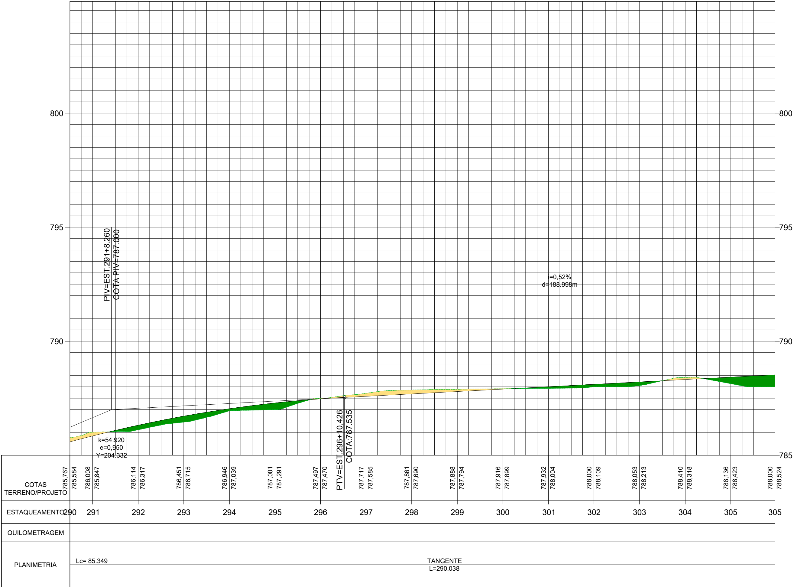
PERFIL - 11 ESC H= 1:1000 ESC V= 1:100
