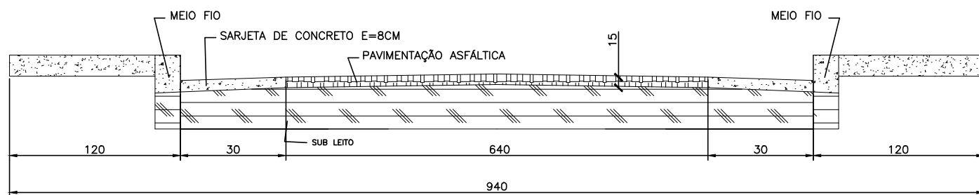
SEÇÃO TRANSVERSAL DA VIA DA ESTACA 19 ATÉ A ESTACA 24 SEM ESCALA
