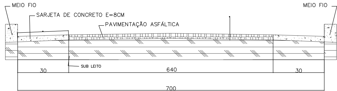
SEÇÃO TRANSVERSAL DA VIA SEM ESCALA
