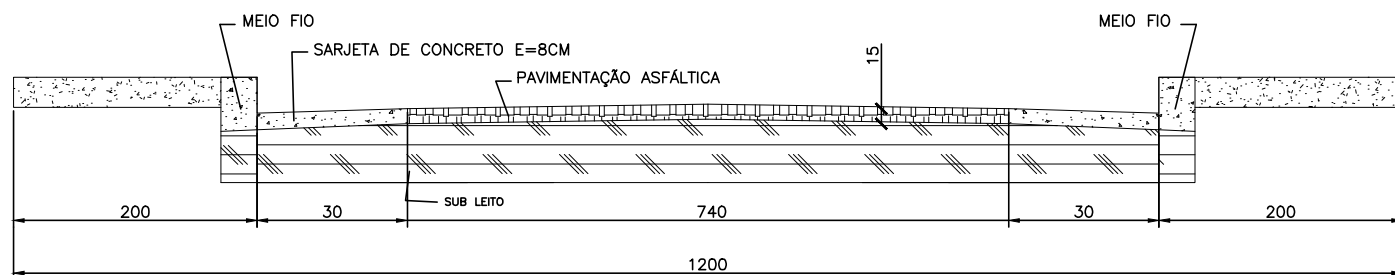
SEÇÃO TRANSVERSAL DA VIA DAS DEMAIS ESTACAS SEM ESCALA
