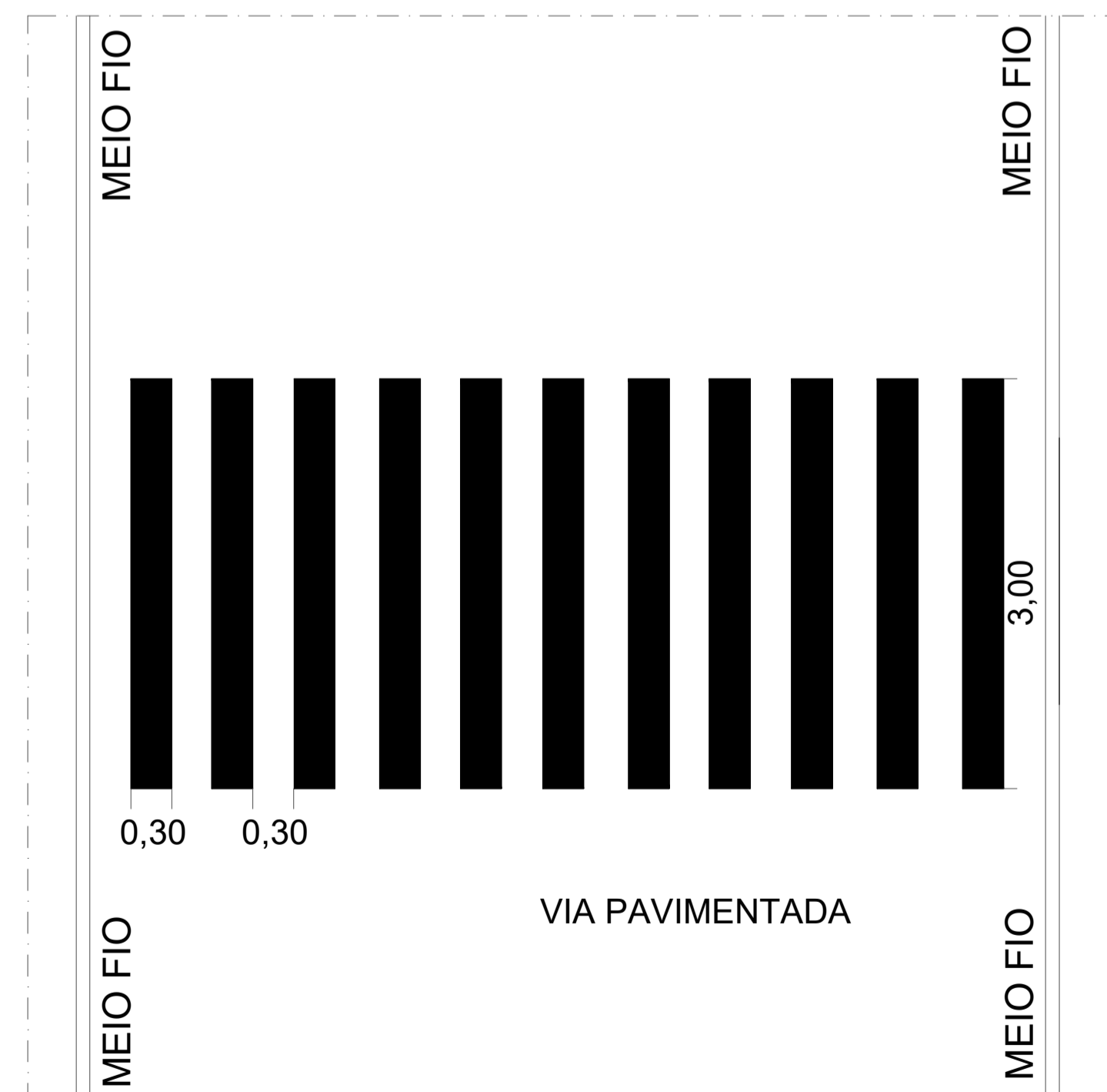
"DETALHE DAS FAIXAS DE PEDESTRE"
