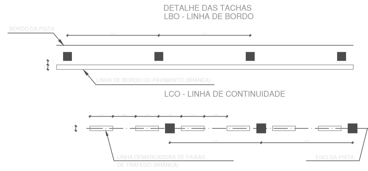
"DETALHE DAS LINHAS E TACHAS"
