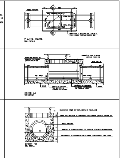
DETALHAMENTO - POÇO DE VISITA
