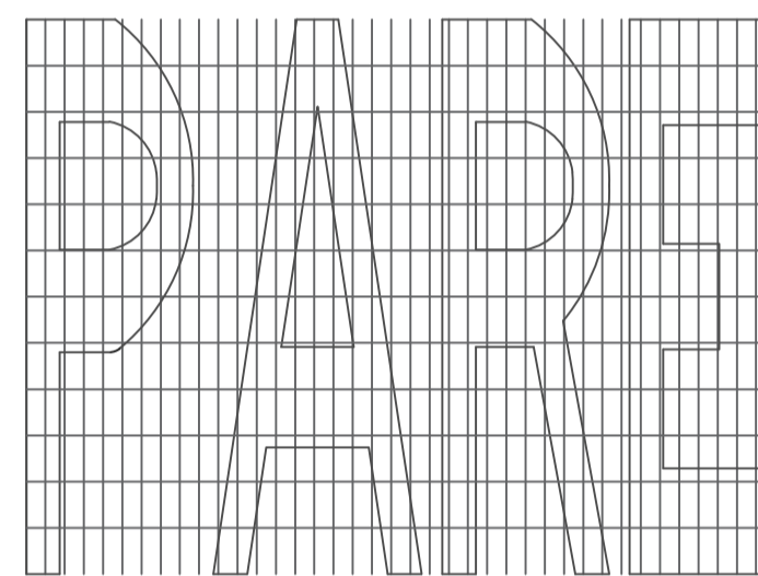
"DETALHE DA DIAGRAMAÇÃO PARE"
