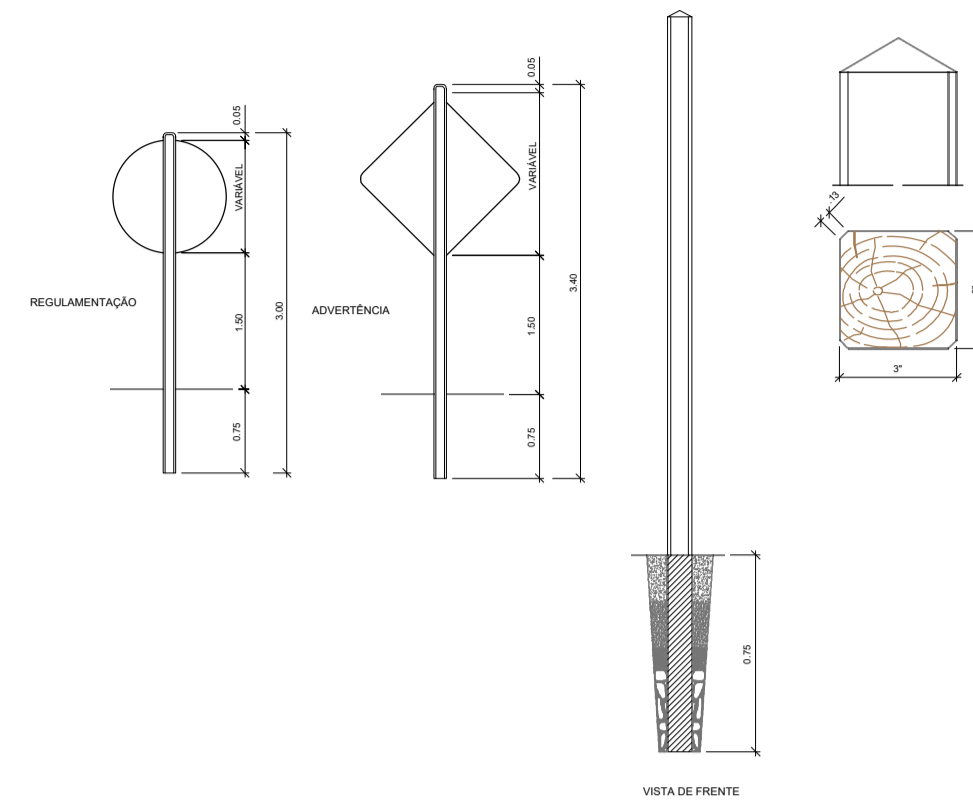
"DETALHE DAS PLACAS"
