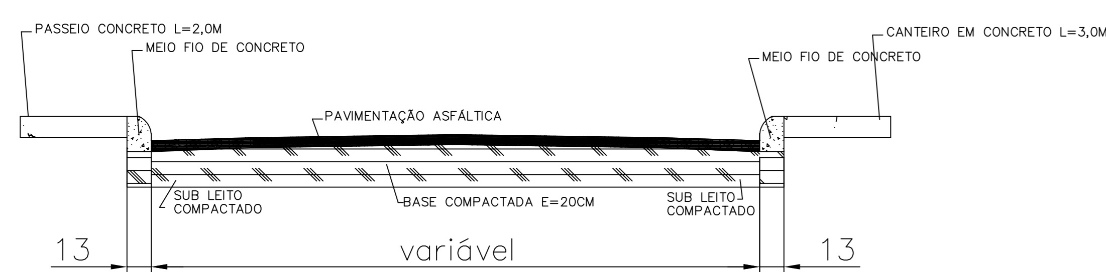
SEÇÃO TRANSVERSAL DA VIA NO TRECHO Sem escala
