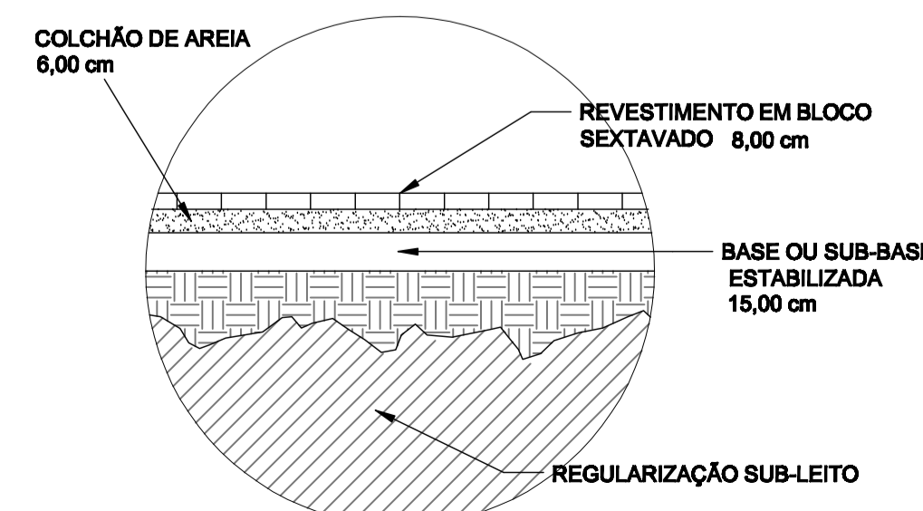
DETALHE 02 CORTE CAMADAS S / ESCALA
