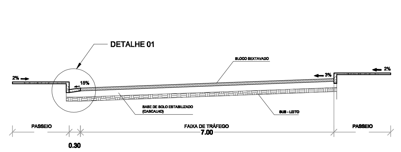
CORTE TRANSVERSAL B - B PISTA DE ROLAMENTO ESCALA - 1/50 RUA PRINCESA ISABEL RUA RACHEL DE QUEIROZ
