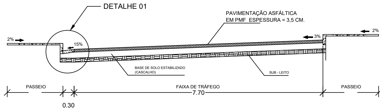
CORTE TRANSVERSAL B - B PISTA DE ROLAMENTO ESCALA - 1/50
