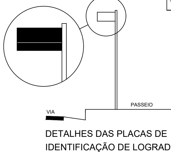
DETALHES PARA LOCAÇÃO DE PLACAS
