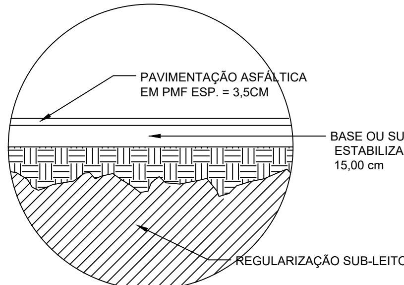
DETALHE 02 CORTE CAMADAS S / ESCALA
