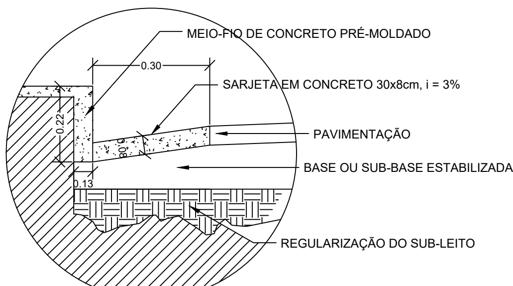
DETALHE 01 MEIO FIO E SARJETAS S / ESCALA
