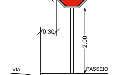
DETALHES PARA LOCAÇÃO DE PLACAS
