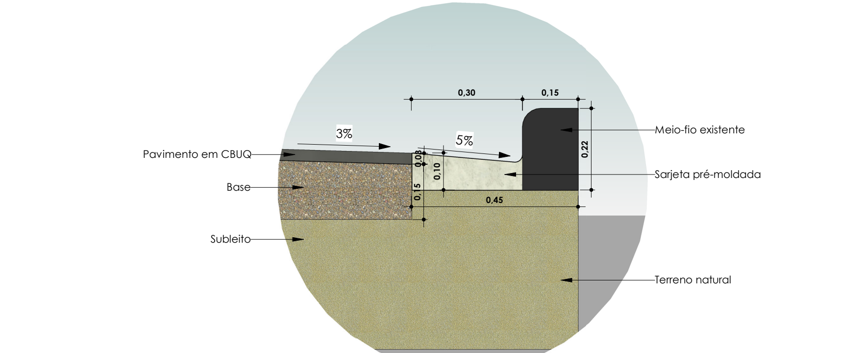
DETALHE MEIO-FIO E SARJETA
