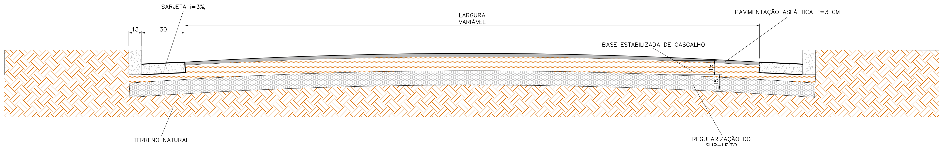
9 CORTE TRANSVERSAL DE RUAS DIVERSAS ESCALA 1:20
