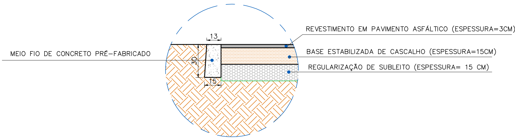
8 DETALHE MEIO FIO DE TRAVAMENTO ESCALA 1:20
