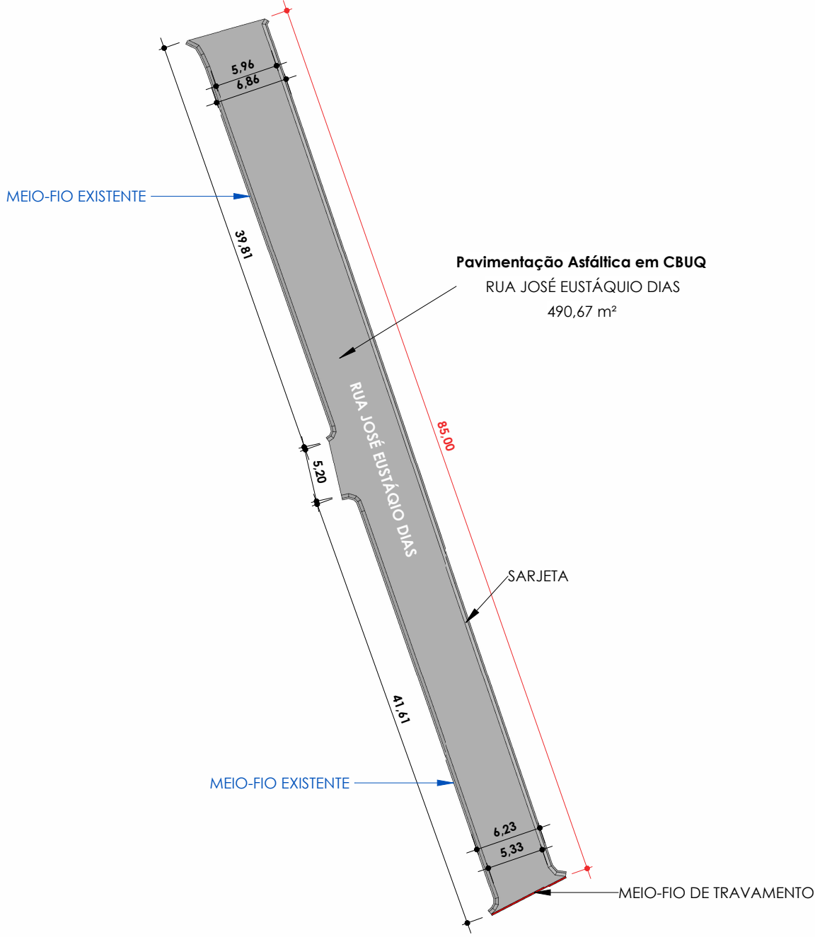
PLANTA DE COTAS - RUA JOSÉ EUSTÁQUIO DIAS ESC: 1 : 500
