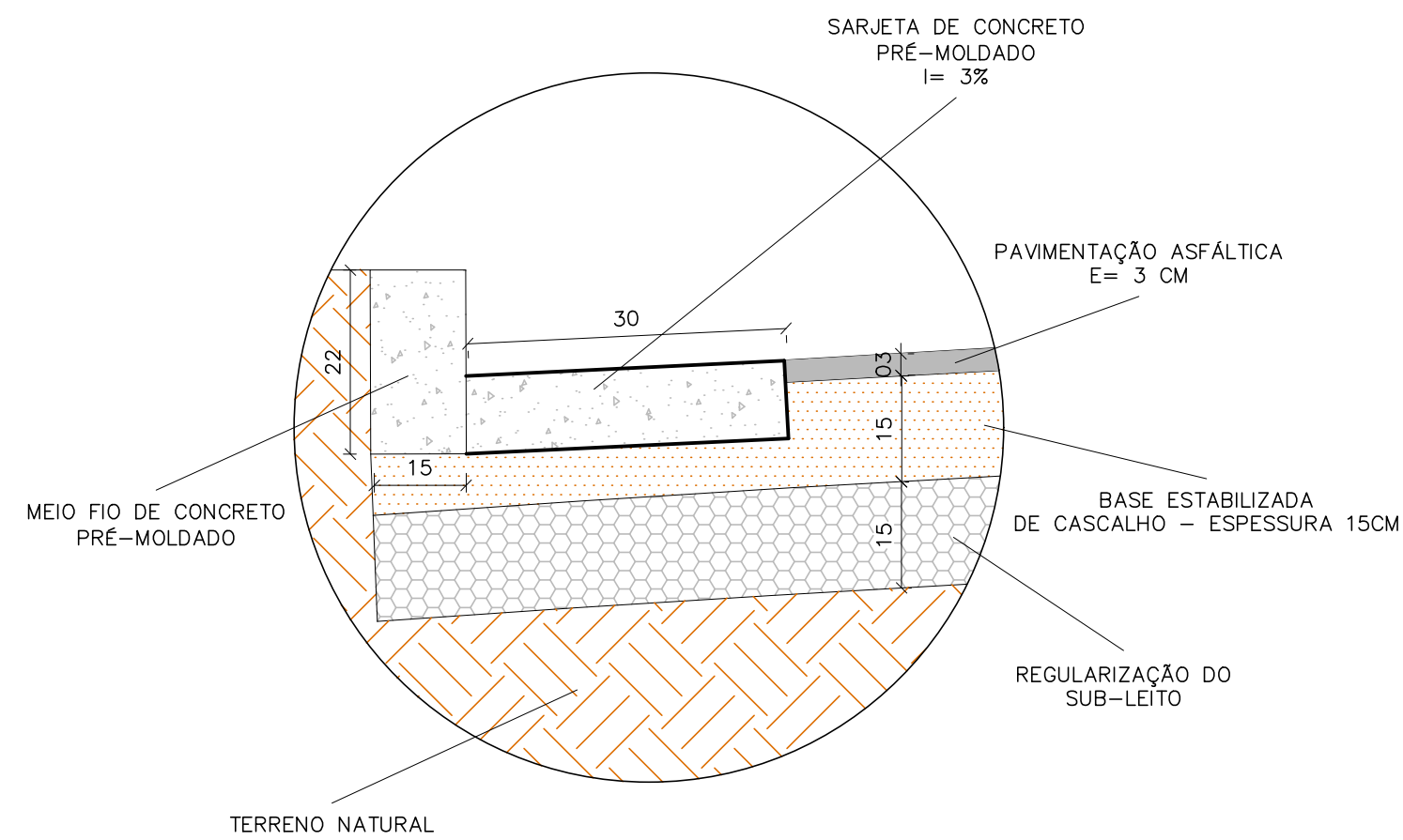
7 DETALHE DA SARJETA E DO MEIO FIO DE RUAS DIVERSAS ESCALA 1:10
