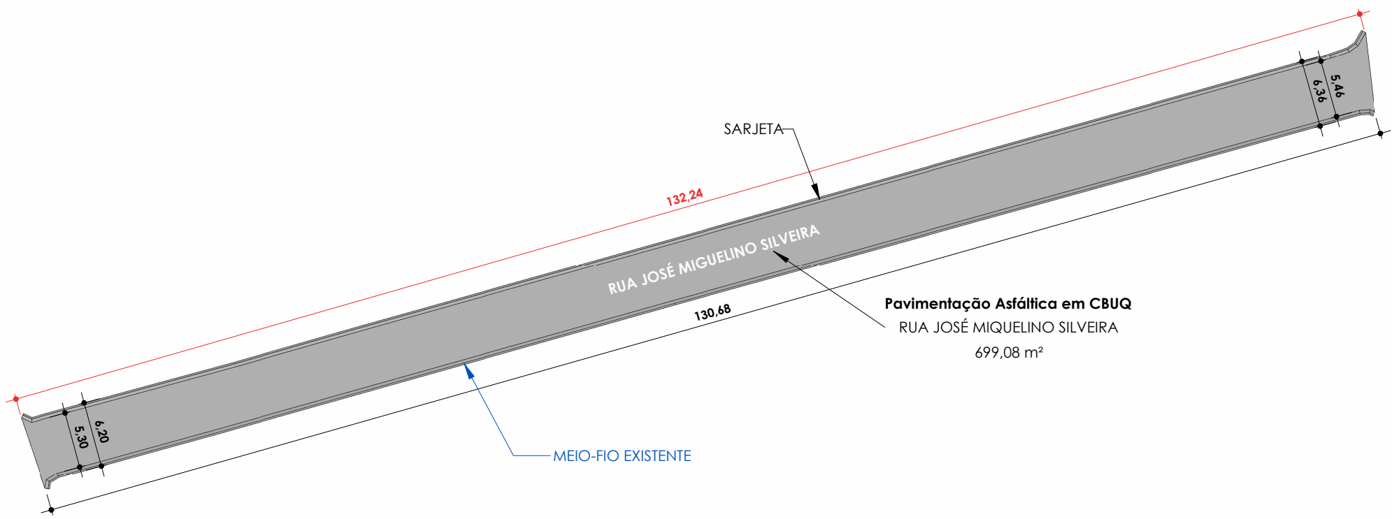
PLANTA DE COTAS - RUA MIQUELINO SILVEIRA ESC: 1 : 500
