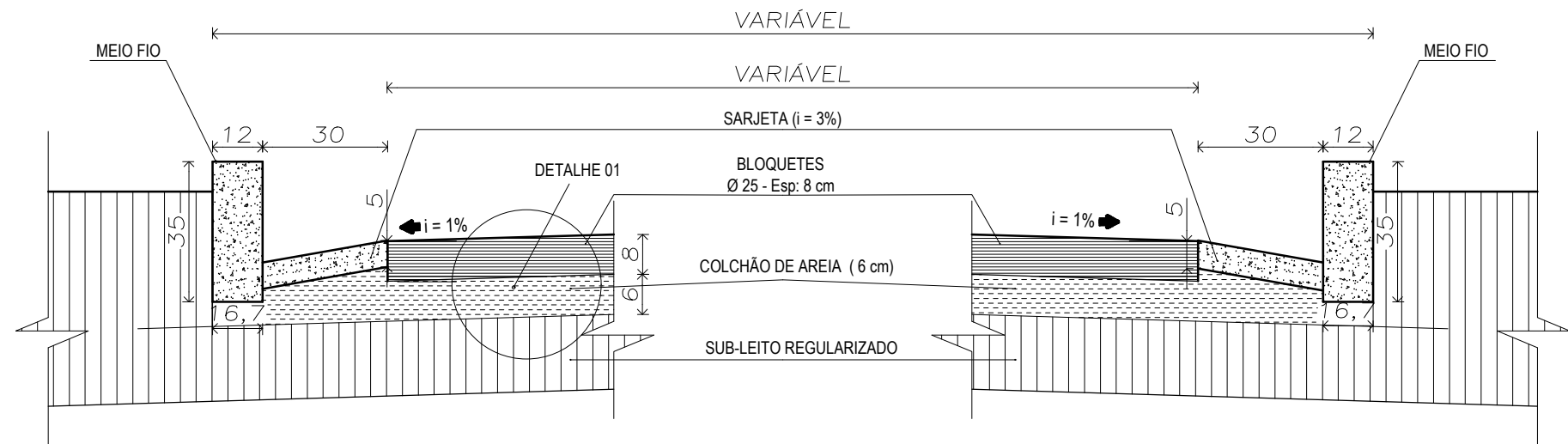
SEÇÃO TRANSVERSAL S/ ESCALA
