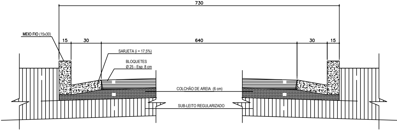
SECÇÃO ESQUEMÁTICA T16 S/ESCALA
