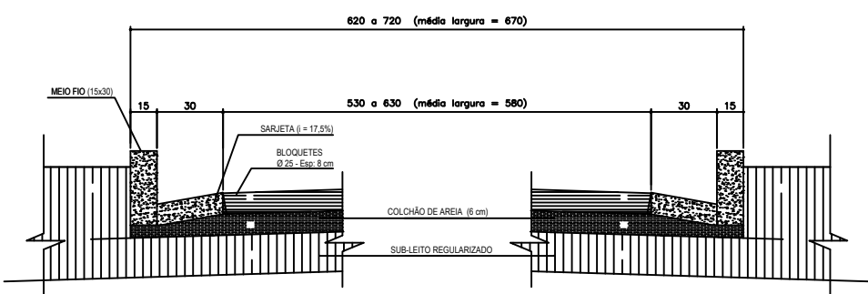
SECÇÃO ESQUEMÁTICA T23
