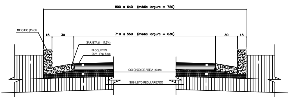
SECÇÃO ESQUEMÁTICA T21
