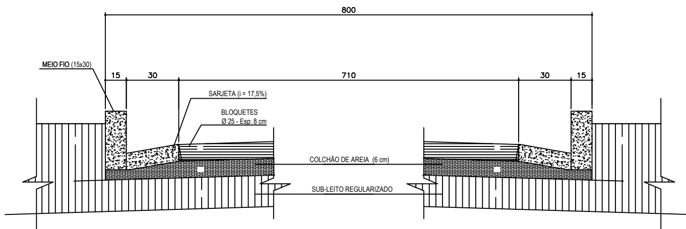
SECÇÃO ESQUEMÁTICA T20
