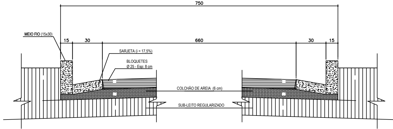
SECÇÃO ESQUEMÁTICA T17 S/ESCALA
