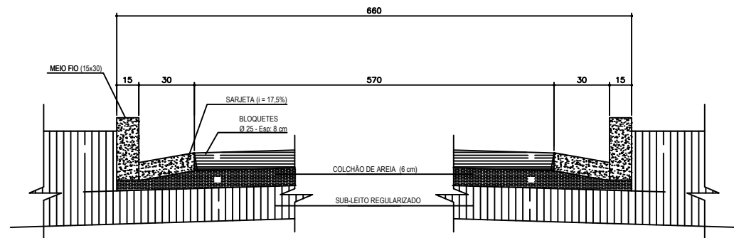
SECÇÃO ESQUEMÁTICA T8 S/ESCALA
