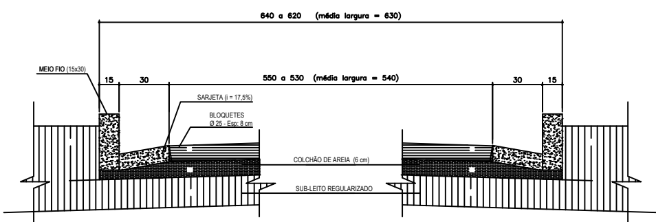
SECÇÃO ESQUEMÁTICA T22
