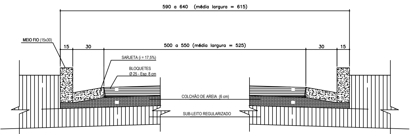
SECÇÃO ESQUEMÁTICA T4 S/ESCALA
