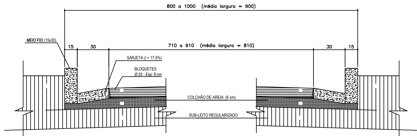
SECÇÃO ESQUEMÁTICA T2 S/ESCALA
