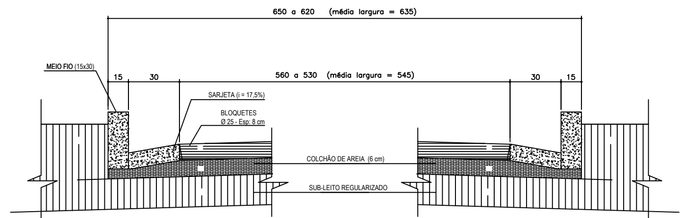
SECÇÃO ESQUEMÁTICA T6 S/ESCALA
