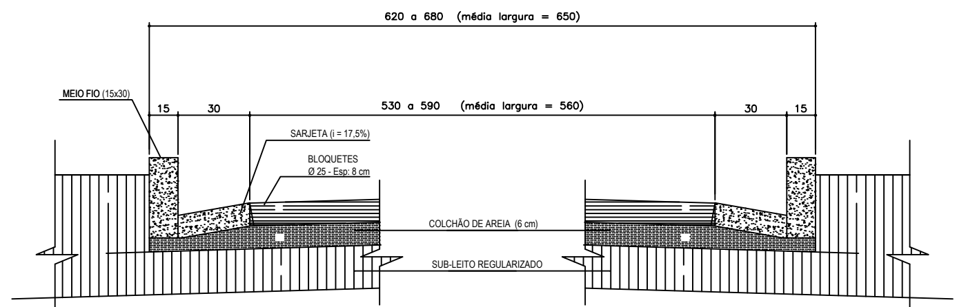
SECÇÃO ESQUEMÁTICA T7 S/ESCALA
