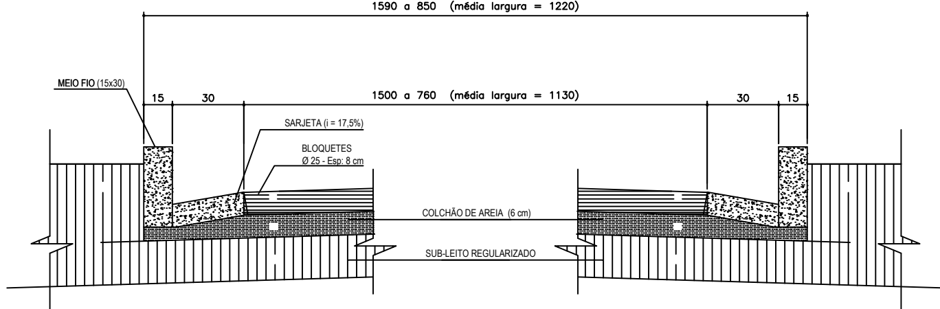
SECÇÃO ESQUEMÁTICA T14 S/ESCALA
