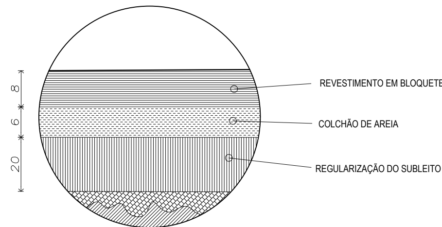
DETALHE 01 - CORTE CAMADAS - BLOQUETE S/ ESCALA
