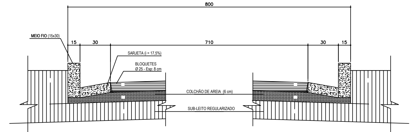
SECÇÃO ESQUEMÁTICA T1 S/ESCALA
