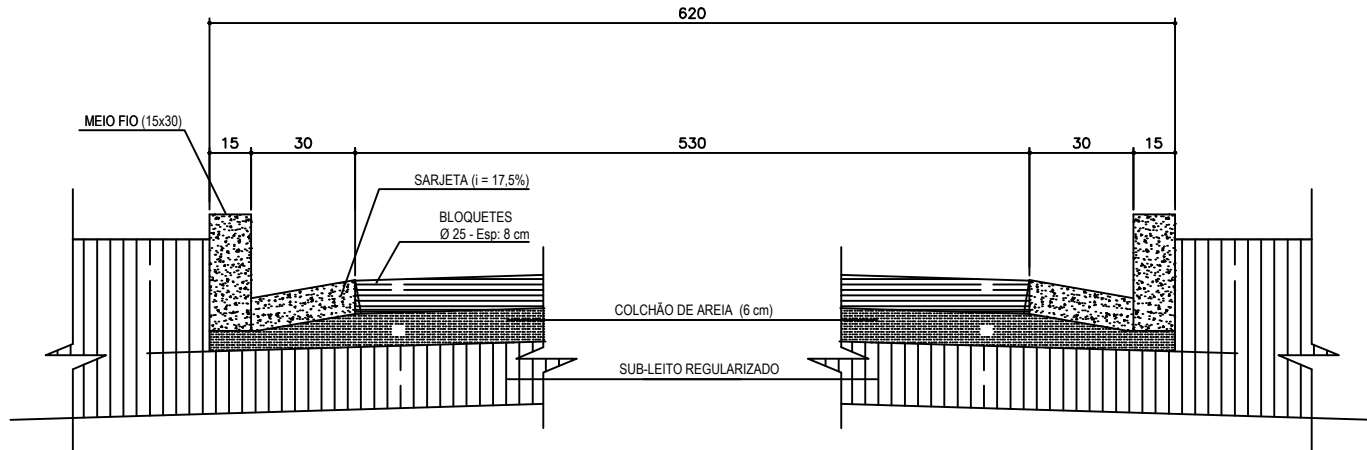
SECÇÃO ESQUEMÁTICA T13 S/ESCALA
