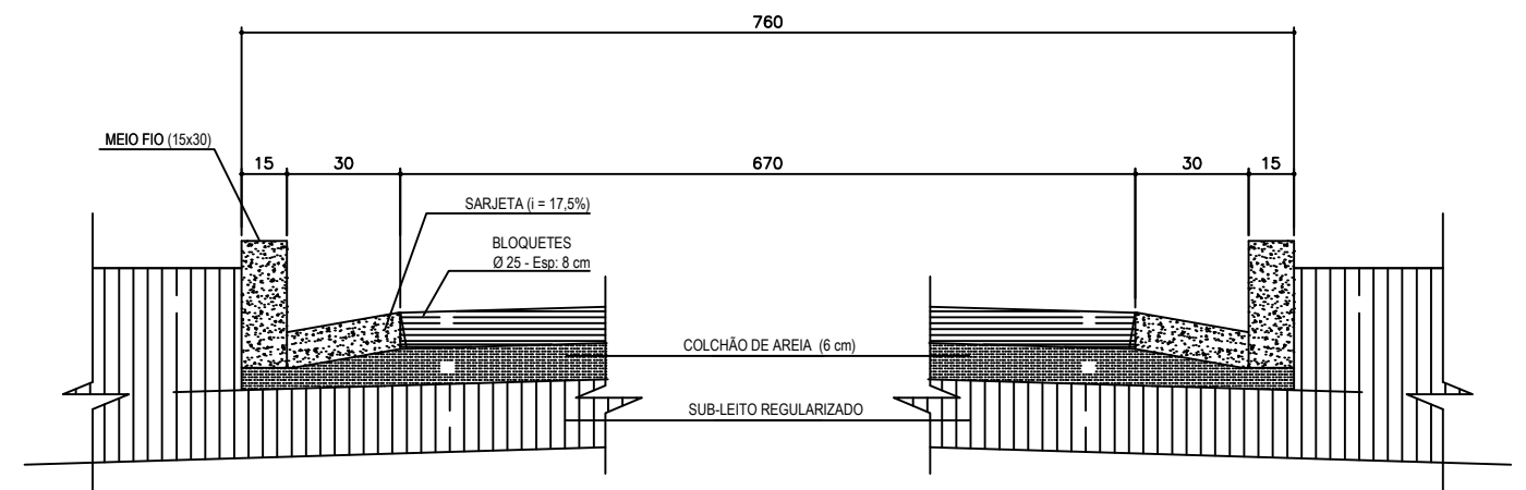
SECÇÃO ESQUEMÁTICA T5 S/ESCALA
