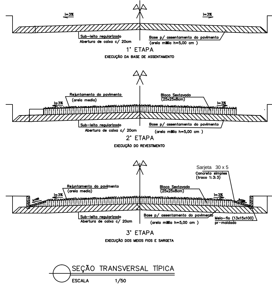
SEÇÃO TRANSVERSAL TÍPICA ESCALA 1/50
