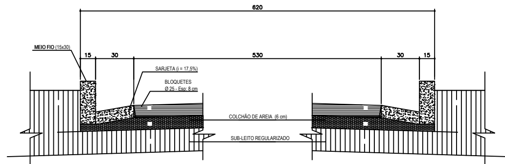
SECÇÃO ESQUEMÁTICA T10 S/ESCALA
