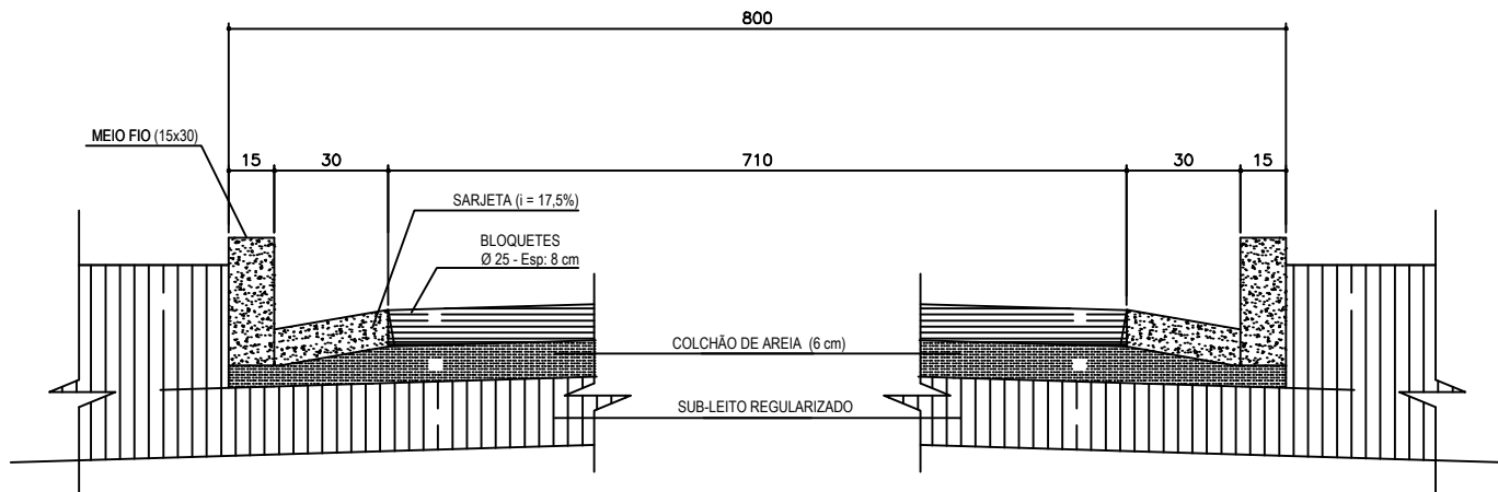
SECÇÃO ESQUEMÁTICA T1 S/ESCALA
