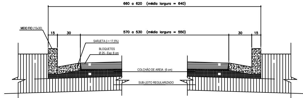
SECÇÃO ESQUEMÁTICA T9 S/ESCALA
