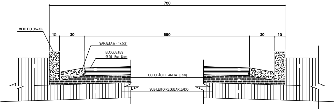
SECÇÃO ESQUEMÁTICA T18 S/ESCALA
