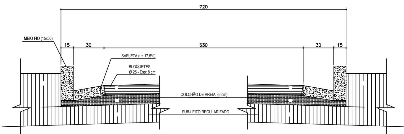
SECÇÃO ESQUEMÁTICA T24
