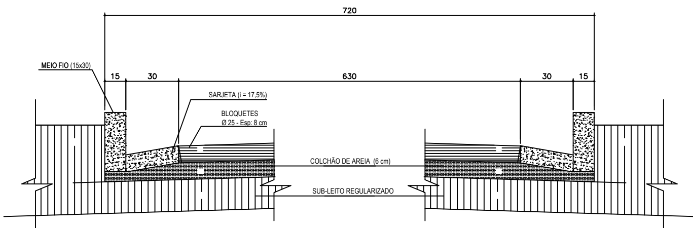
SECÇÃO ESQUEMÁTICA T25
