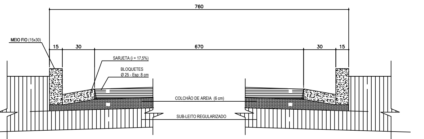
SECÇÃO ESQUEMÁTICA T5 S/ESCALA
