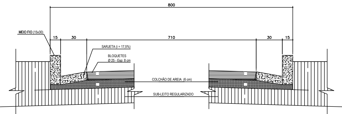
SECÇÃO ESQUEMÁTICA T19
