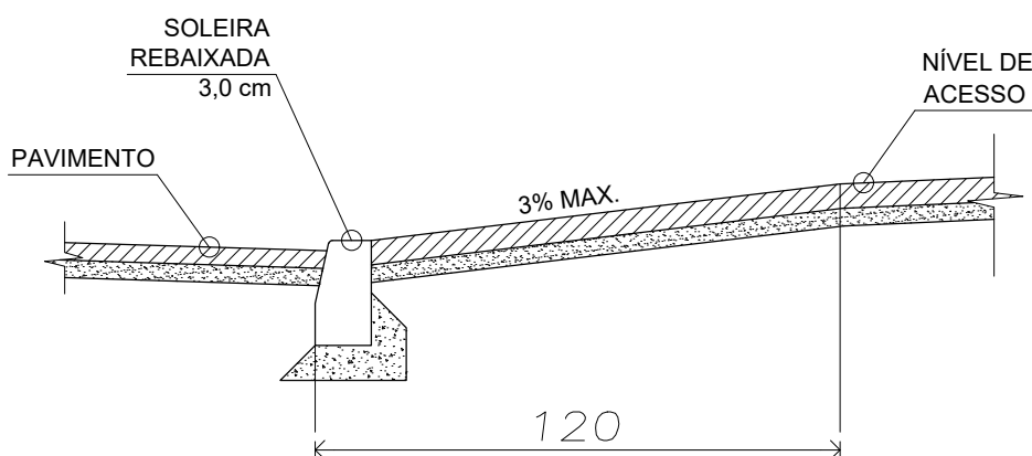
DETALHE - CORTE S/ ESCALA
