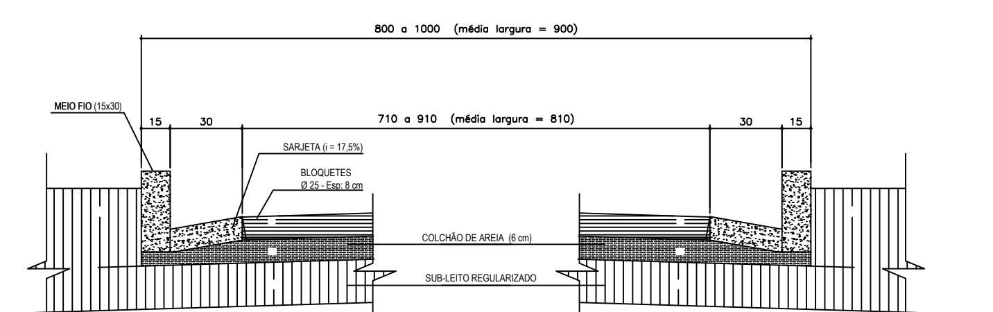
SECÇÃO ESQUEMÁTICA T2 S/ESCALA
