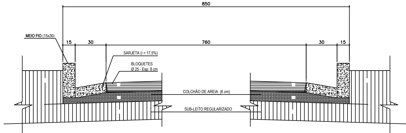
SECÇÃO ESQUEMÁTICA T15 S/ESCALA
