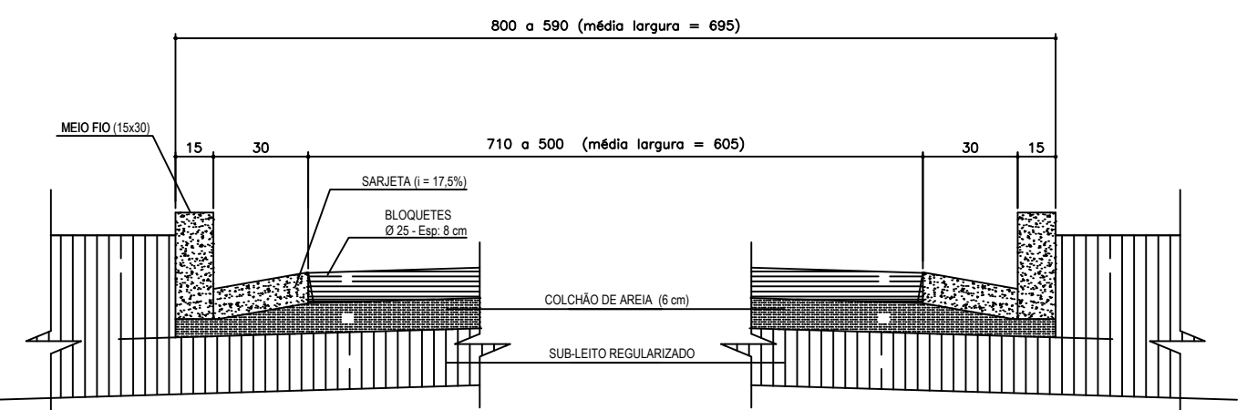
SECÇÃO ESQUEMÁTICA T3 S/ESCALA
