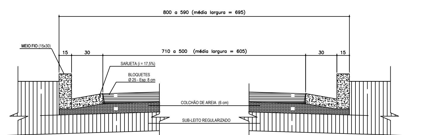
SECÇÃO ESQUEMÁTICA T3 S/ESCALA
