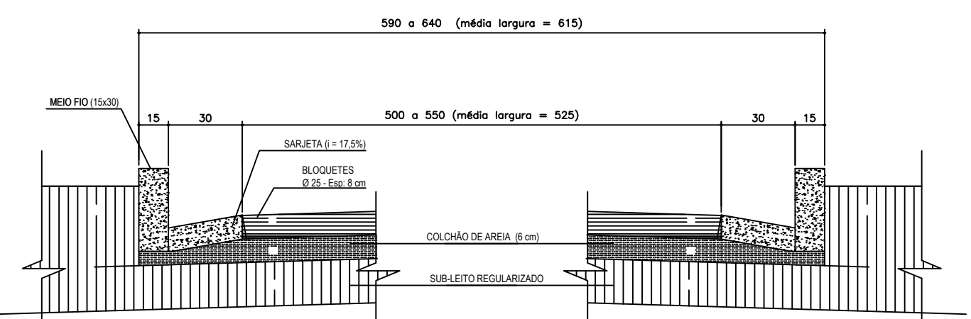
SECÇÃO ESQUEMÁTICA T4 S/ESCALA
