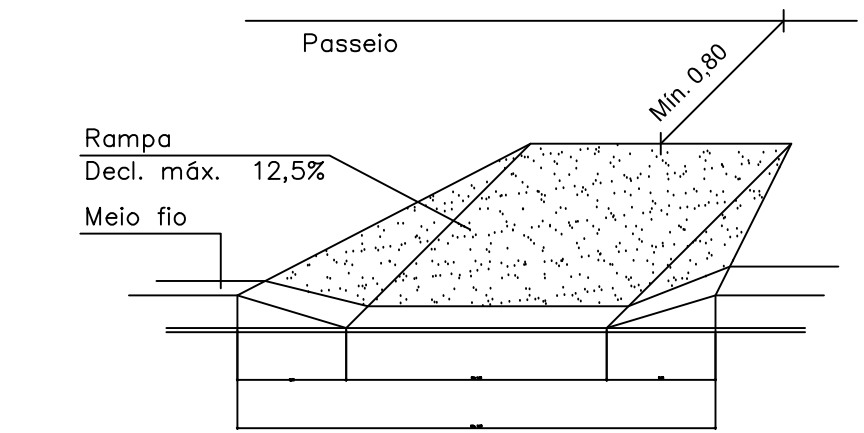
RAMPA (DETALHE 01) S/ ESCALA
