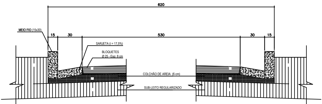
SECÇÃO ESQUEMÁTICA T11 S/ESCALA
