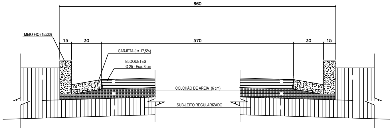
SECÇÃO ESQUEMÁTICA T12 S/ESCALA
