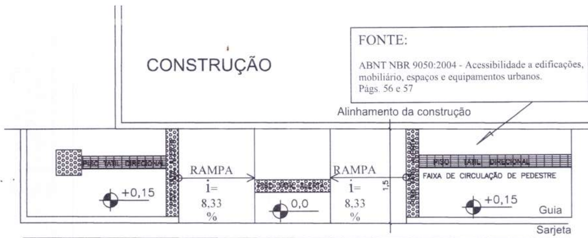
DET. RAMPAS
