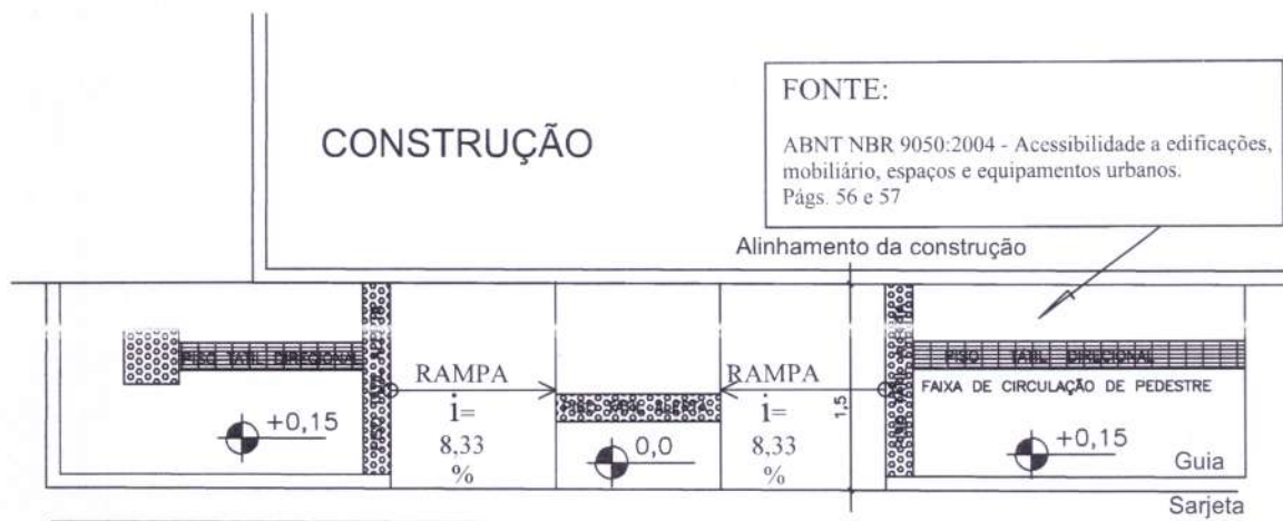
DET. RAMPAS
