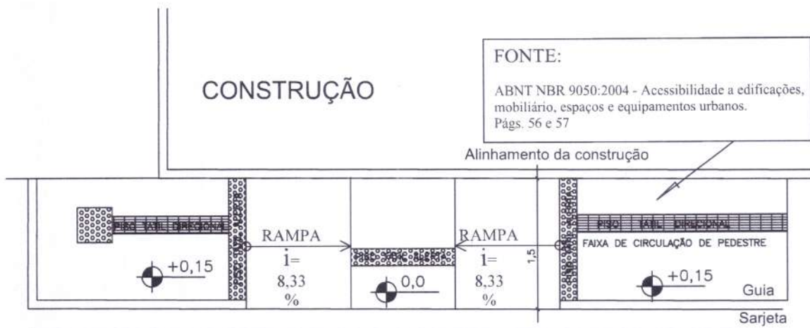
DET. RAMPAS
