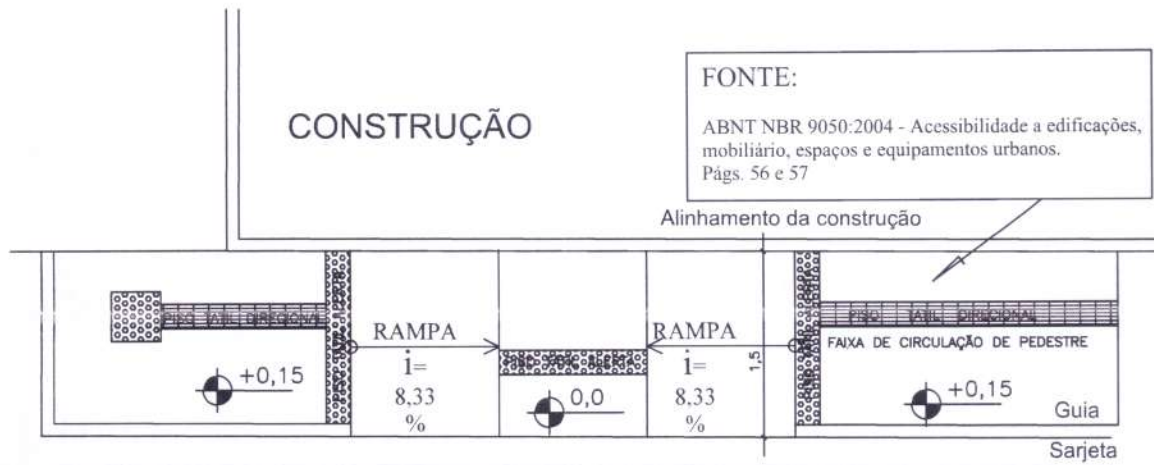
DET. RAMPAS
