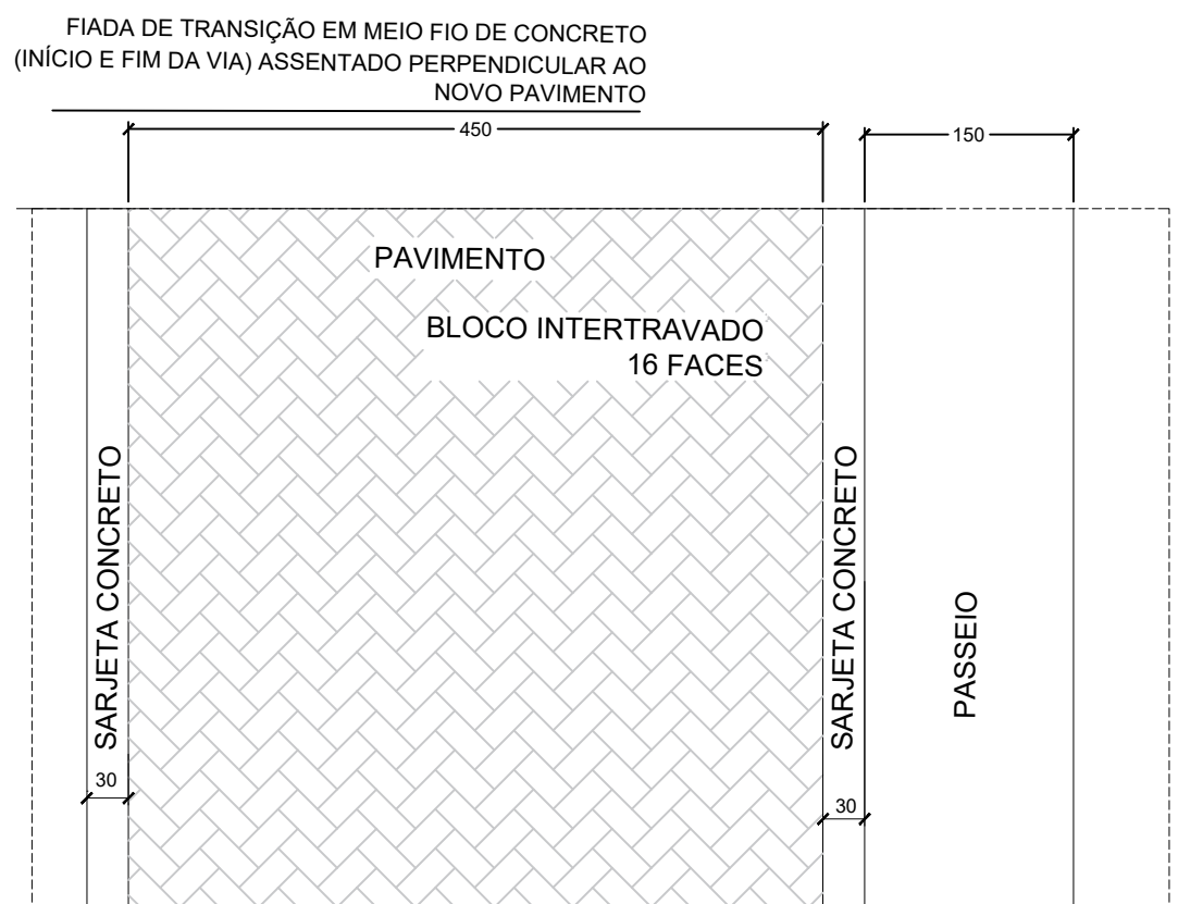
DETALHE 02 - VIA/ SARJETA / PASSEIO ESC 1 --- 50
