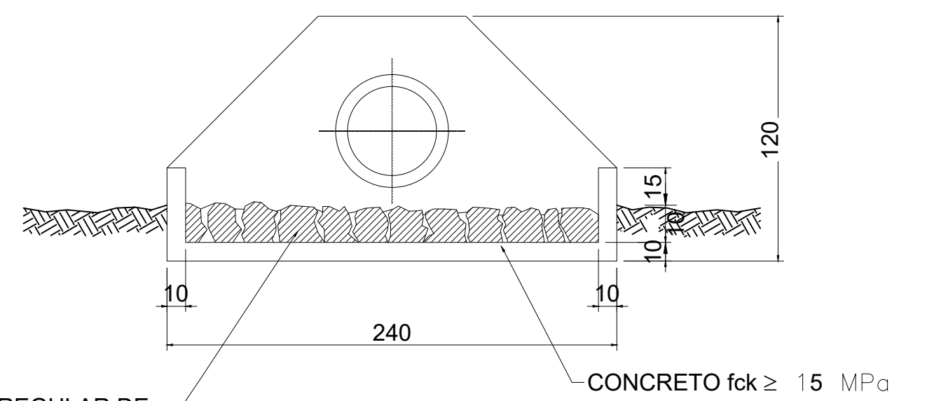
CORTE B-B
