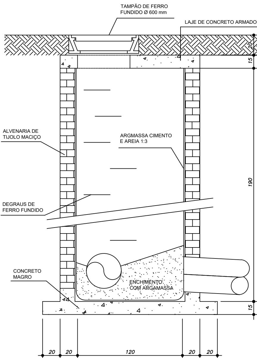
CORTE - A.A
