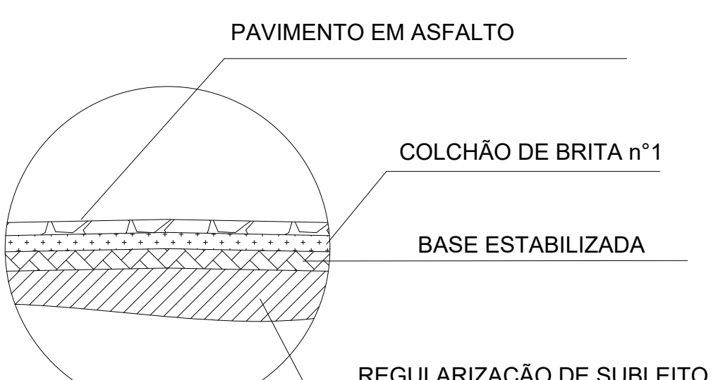
DETALHE 02 - PAVIMENTO ESC 1 --- 50
