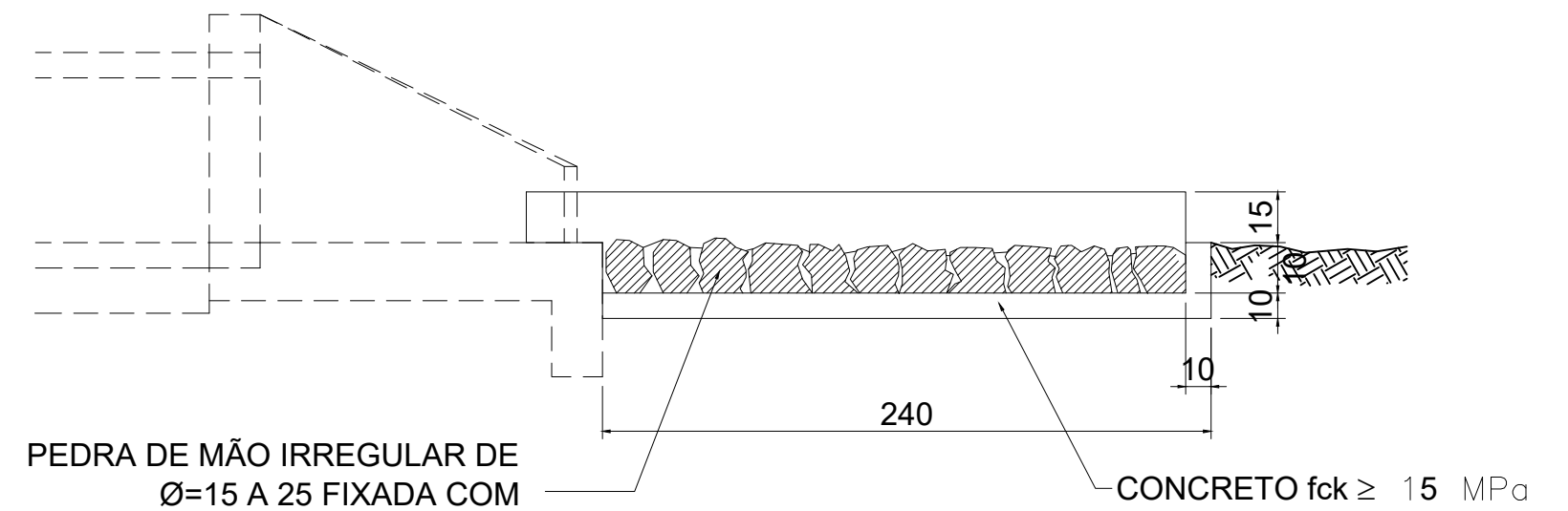
CORTE A-A
