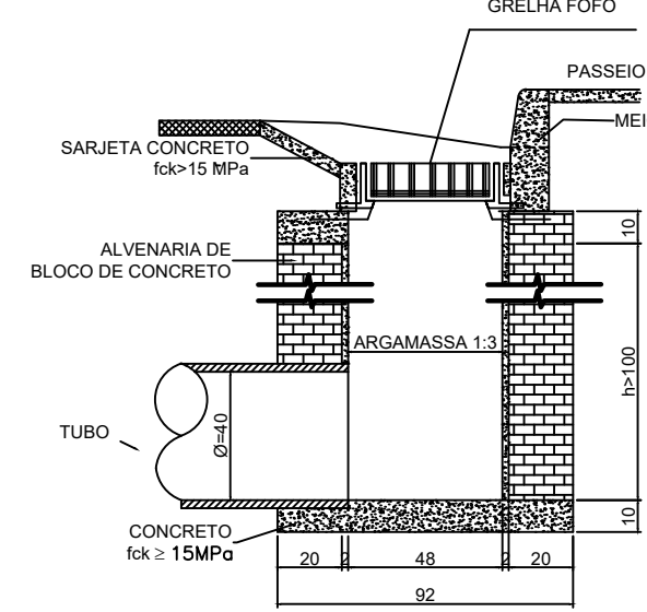
CORTE B-B
