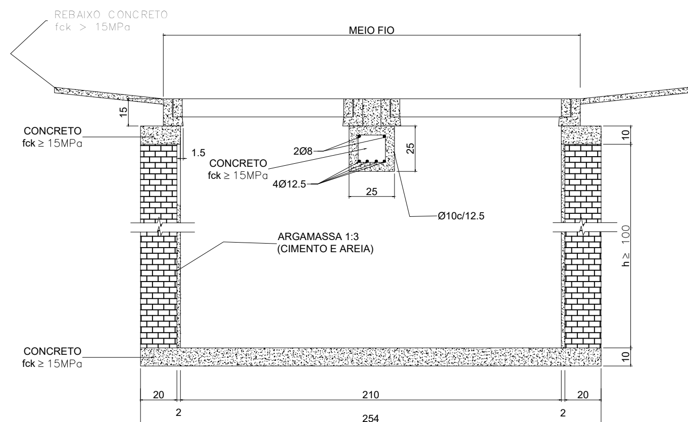
CORTE A-A
