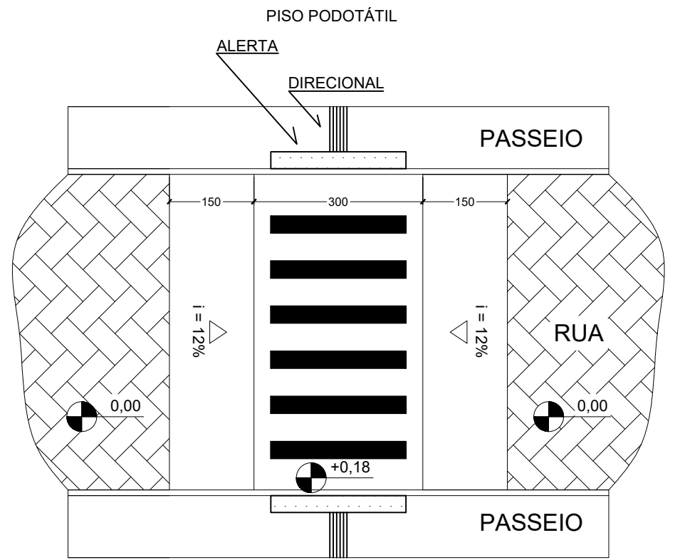
DETALHE 05 - FAIXA ELEVADA ESC 1 --- 75
