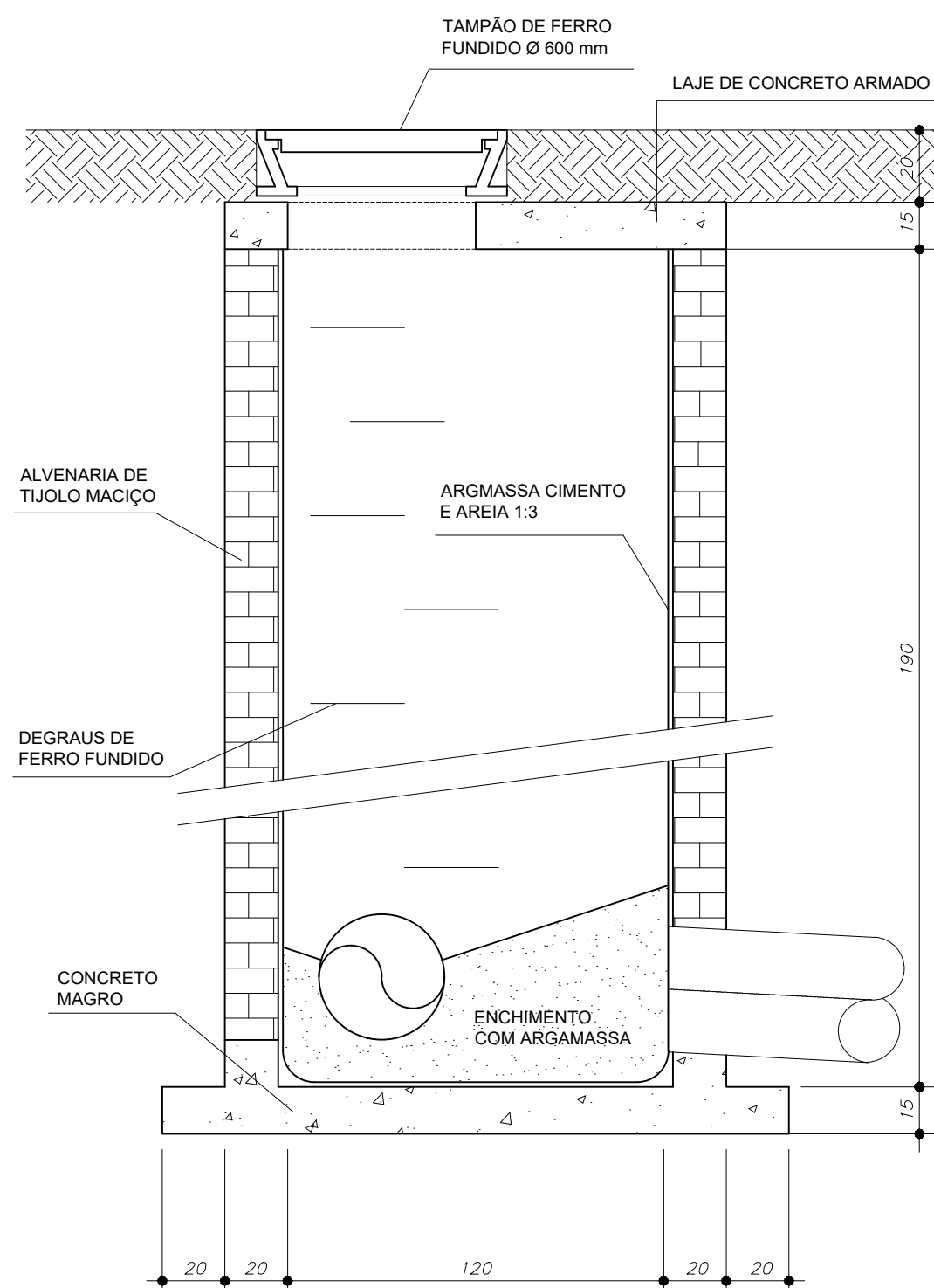
CORTE - A.A
