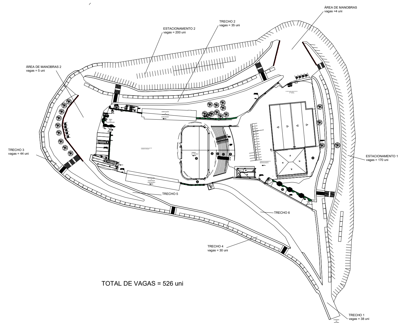
ESTACIONAMENTO ESC 1 --- 2000
