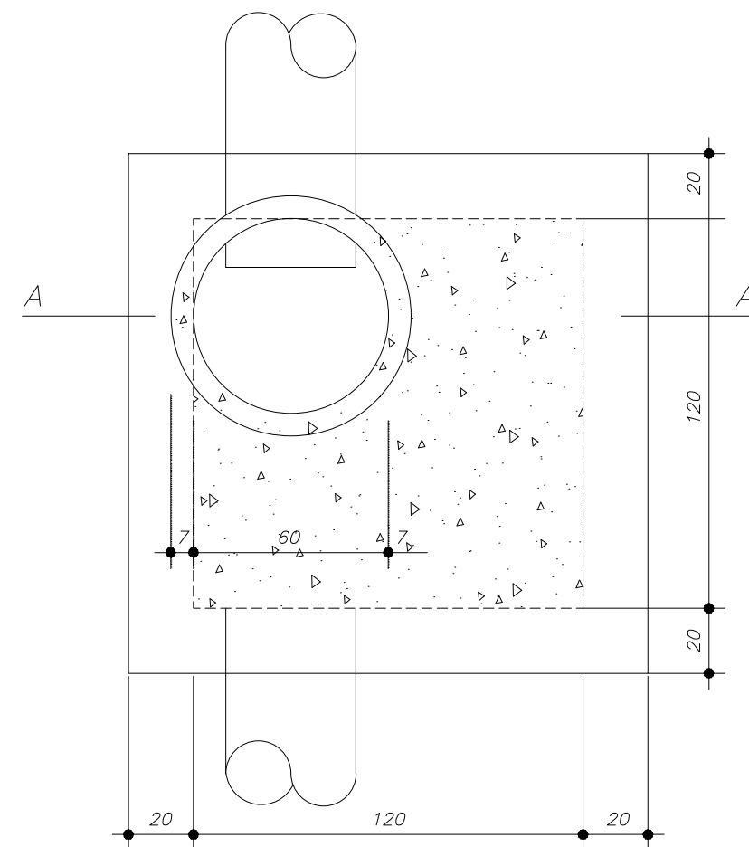
PLANTA
