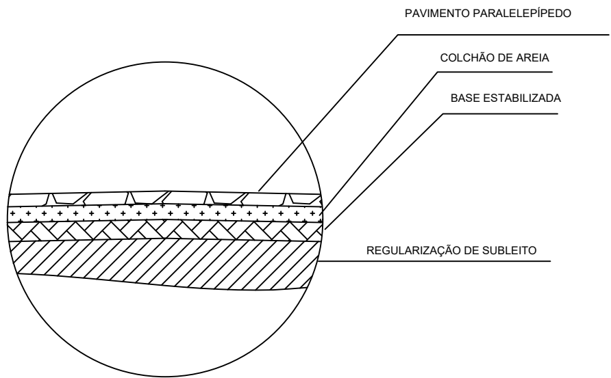
DETALHE 02 - PAVIMENTO ESC 1 --- 20
