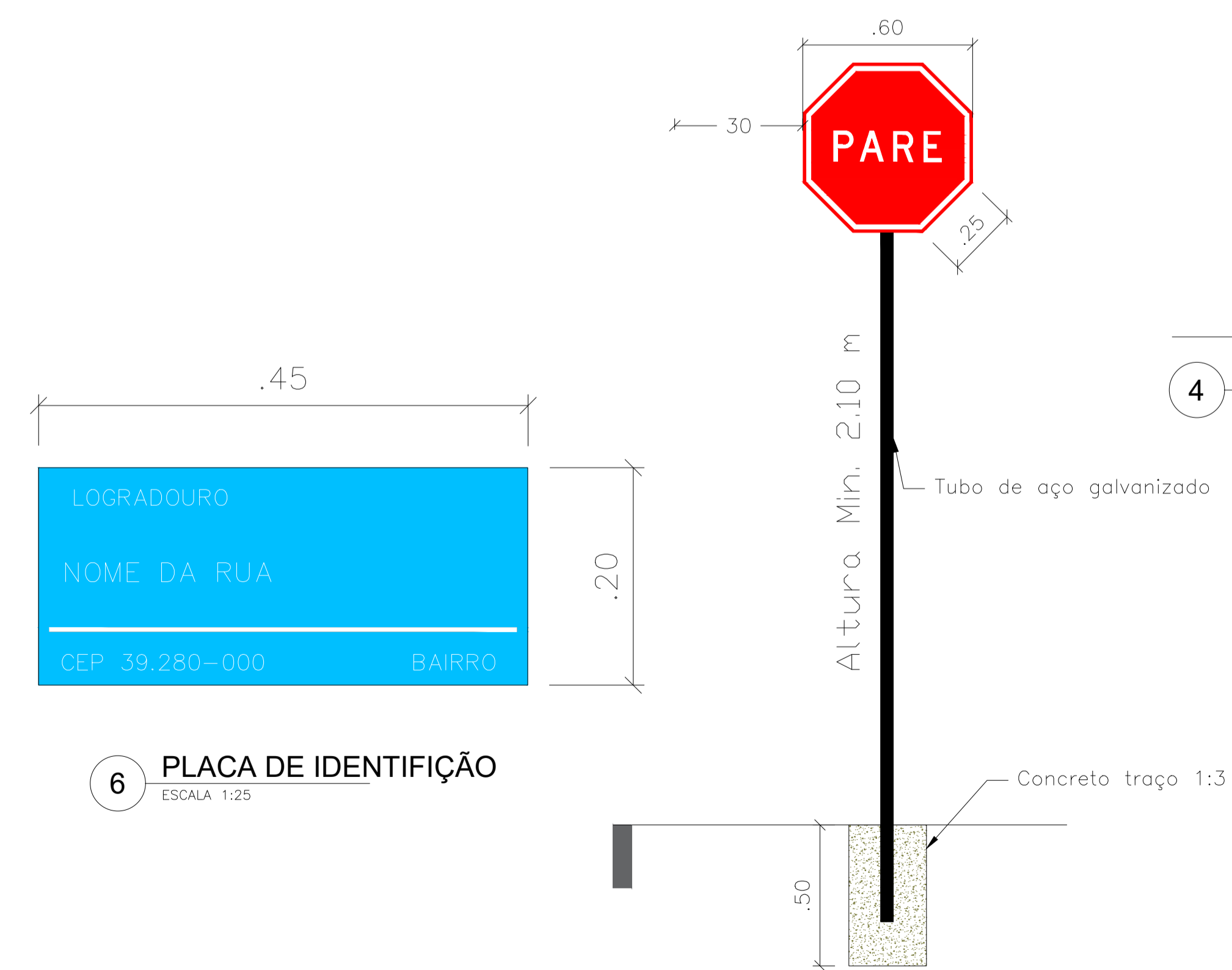
7 DETALHE SINALIZAÇÃO PARE ESCALA 1:25
