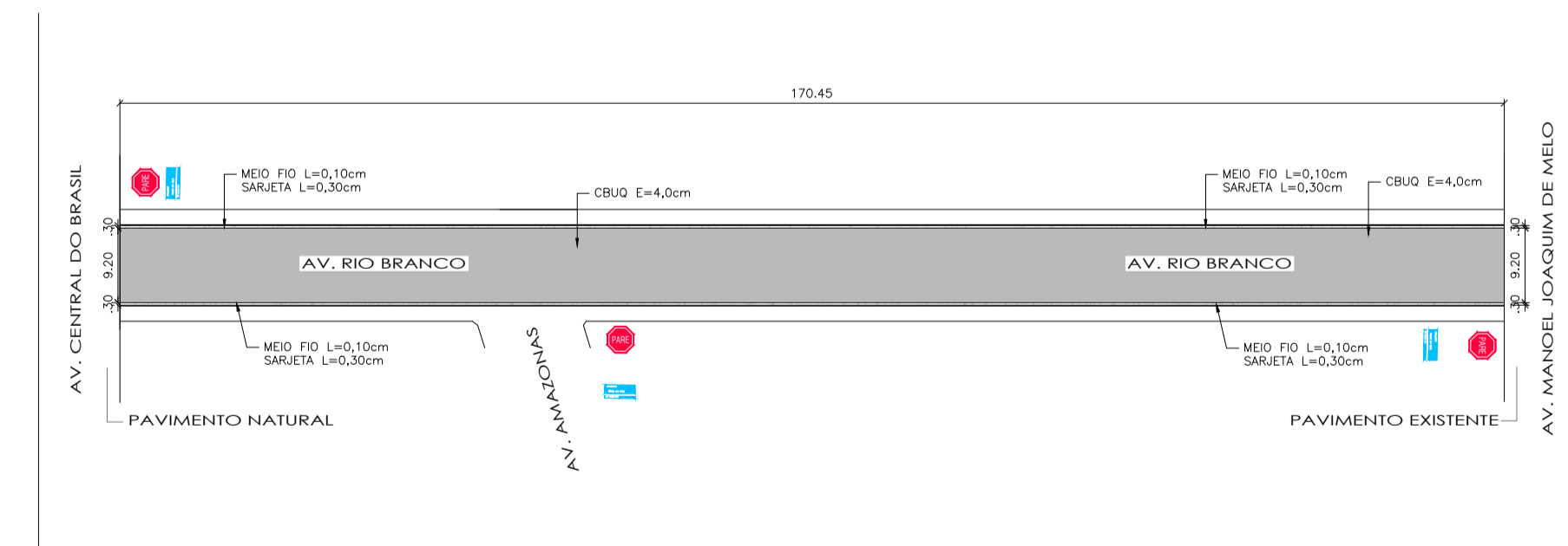
17 PAVIMENTAÇÃO AV. RIO BRANCO ESCALA 1:500
