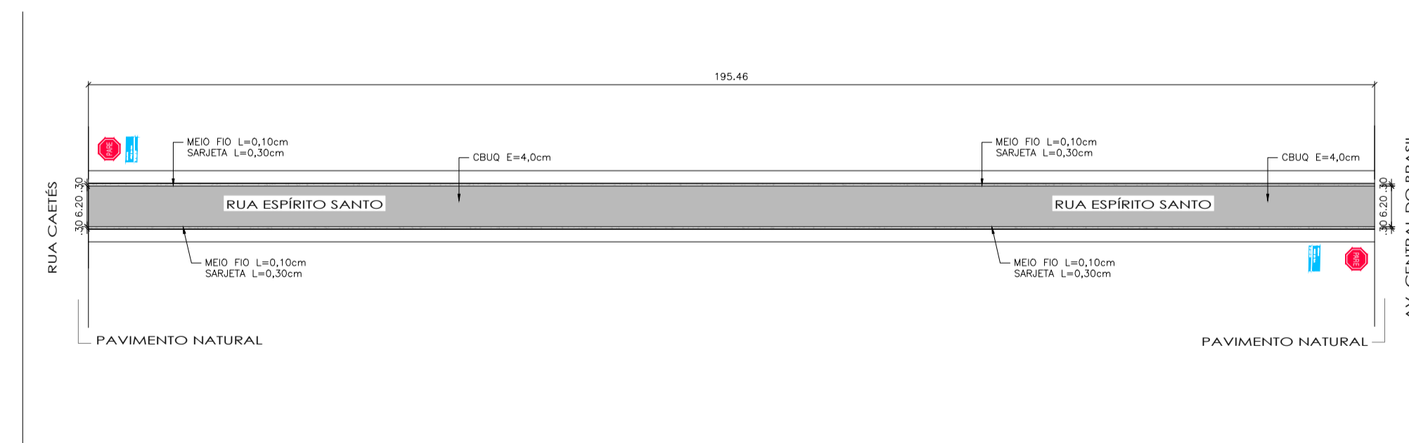
18 PAVIMENTAÇÃO RUA ESPÍRITO SANTO ESCALA 1:500
