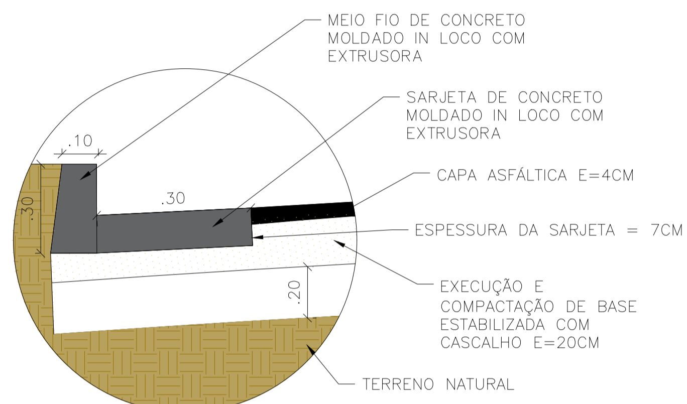
2 DETALHE MEIO FIO E SARJETA ESCALA 1:20
