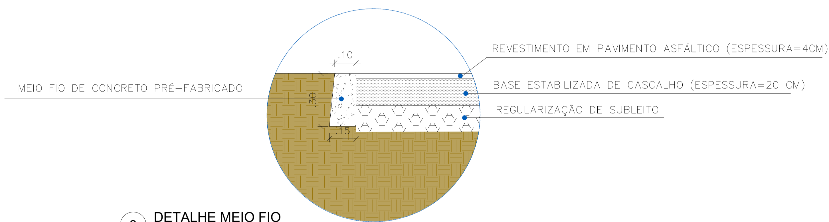
3 DETALHE MEIO FIO ESCALA 1:20
