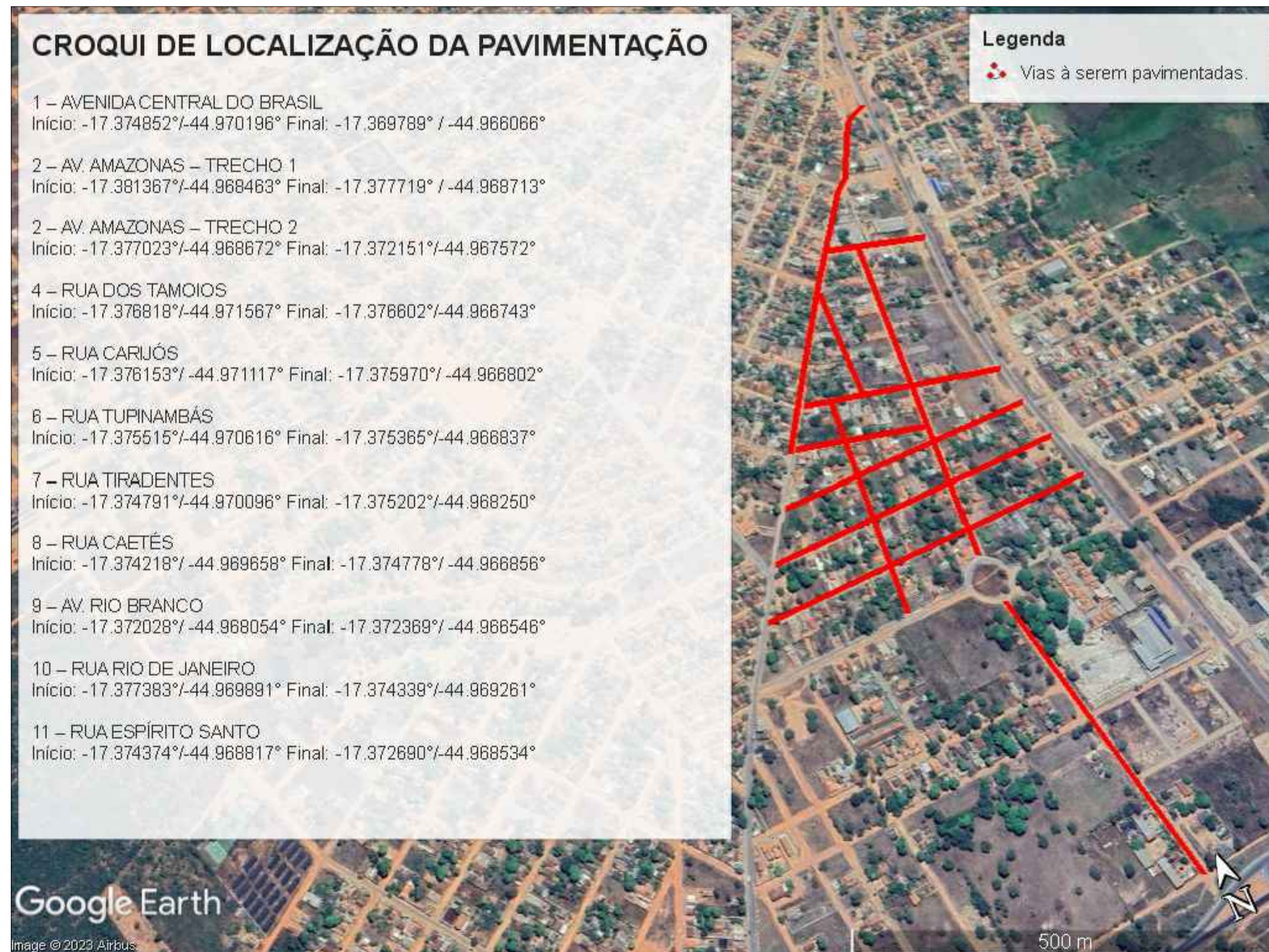
5 LOCALIZAÇÃO SEM ESCALA
