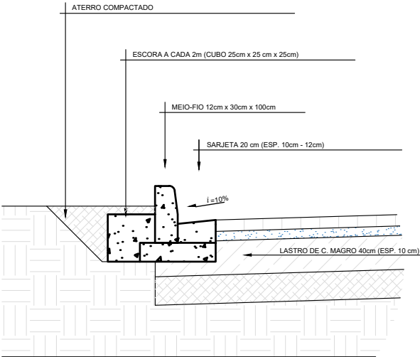
DET. - MEIO-FIO E SARJETA ESCALA 1:20
