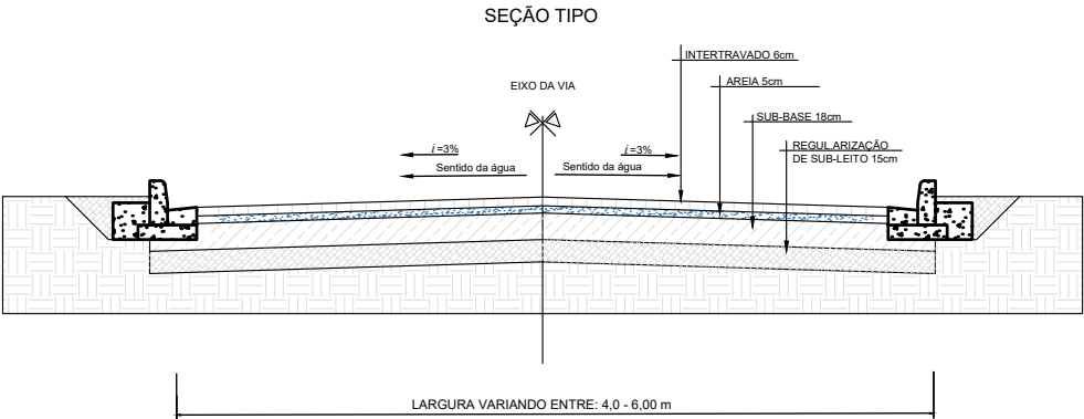
SEÇÃO TIPO - PAVIMENTAÇÃO COM BLOCO INTERTRAVADO ESCALA 1:40
