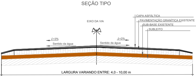
SEÇÃO TIPO - CAPA ASFÁLTICA 1:40
