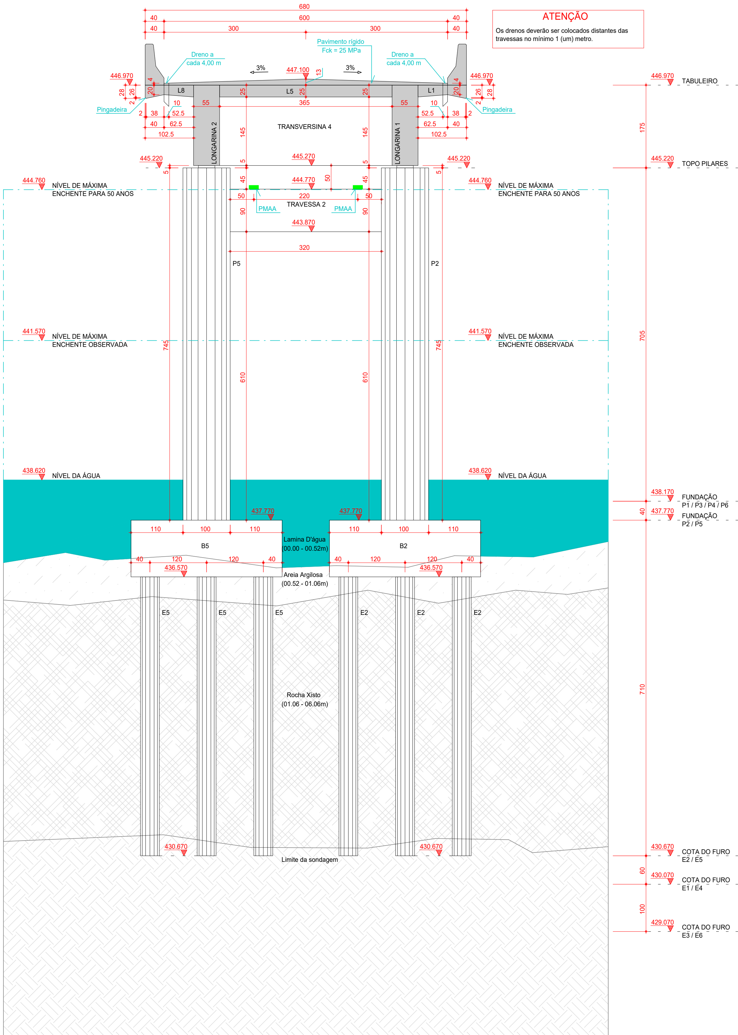
Corte B-B ESC.:1:50
