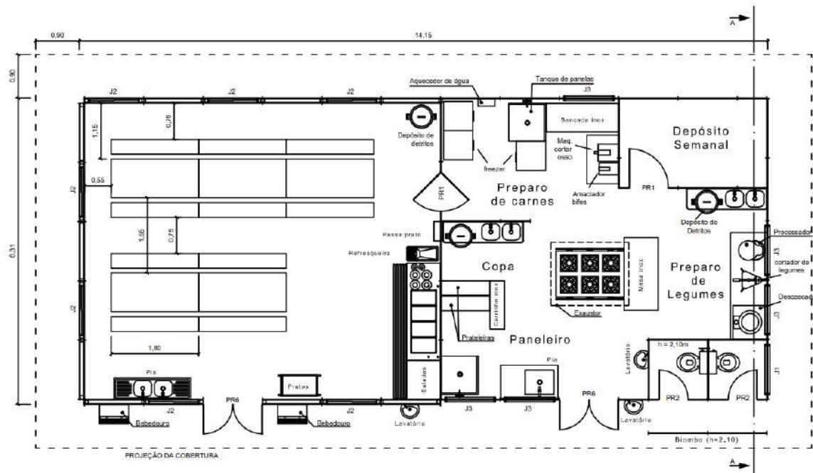
Figura 9 – Refeitório e Cozinha (Obras de Pequeno Porte)
