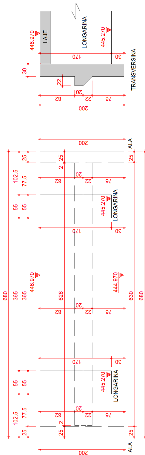
Figura 89 - Geometria transversinas 1 e 7
