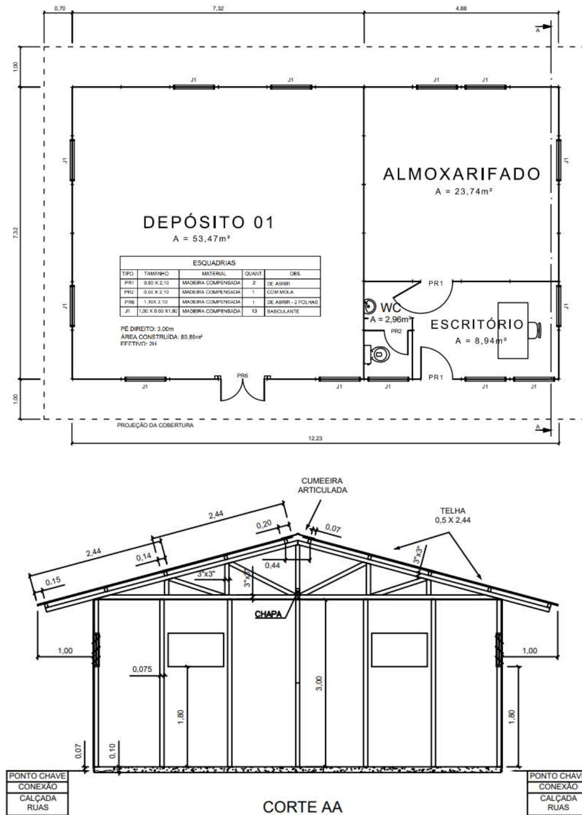
Figura 6 – Almoxarifado (Obras de Pequeno Porte)
