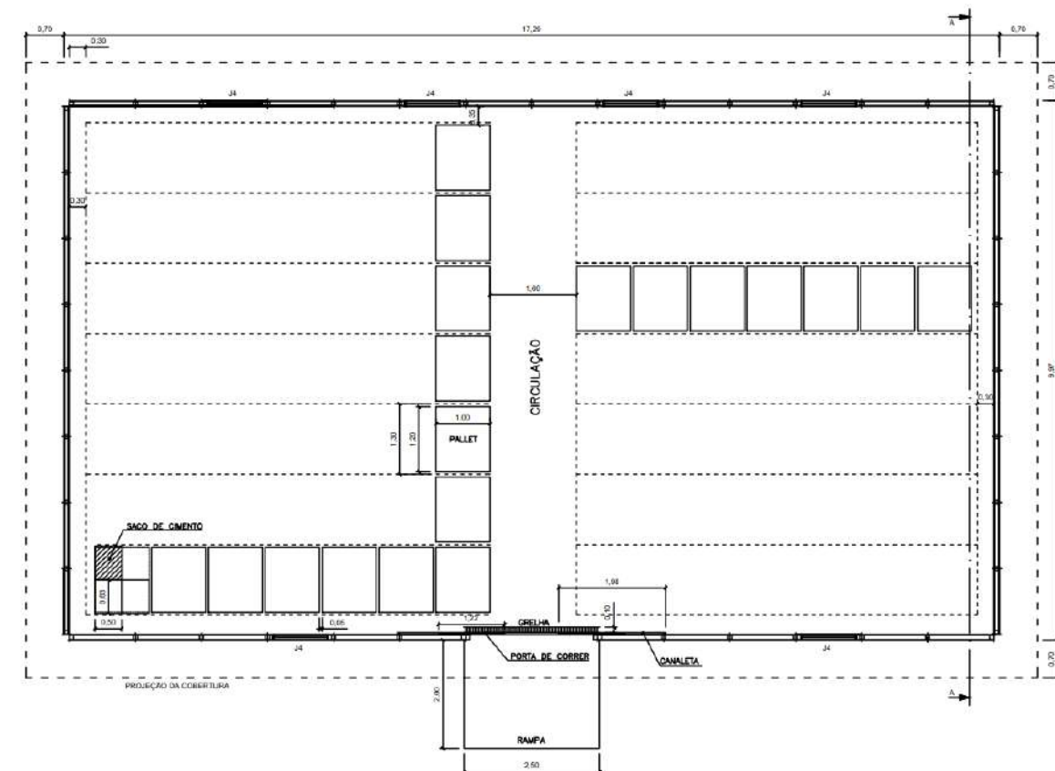
Figura 7 – Depósito de Cimento (Obras de Pequeno Porte)
