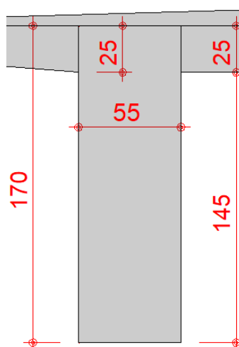
Figura 64 - Seção longarinas
