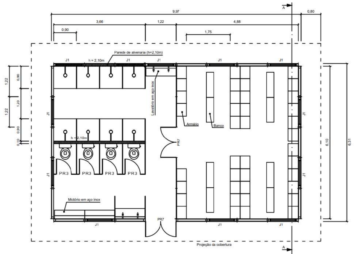
Figura 11 – Banheiro e Vestiário (Obras de Pequeno Porte)
