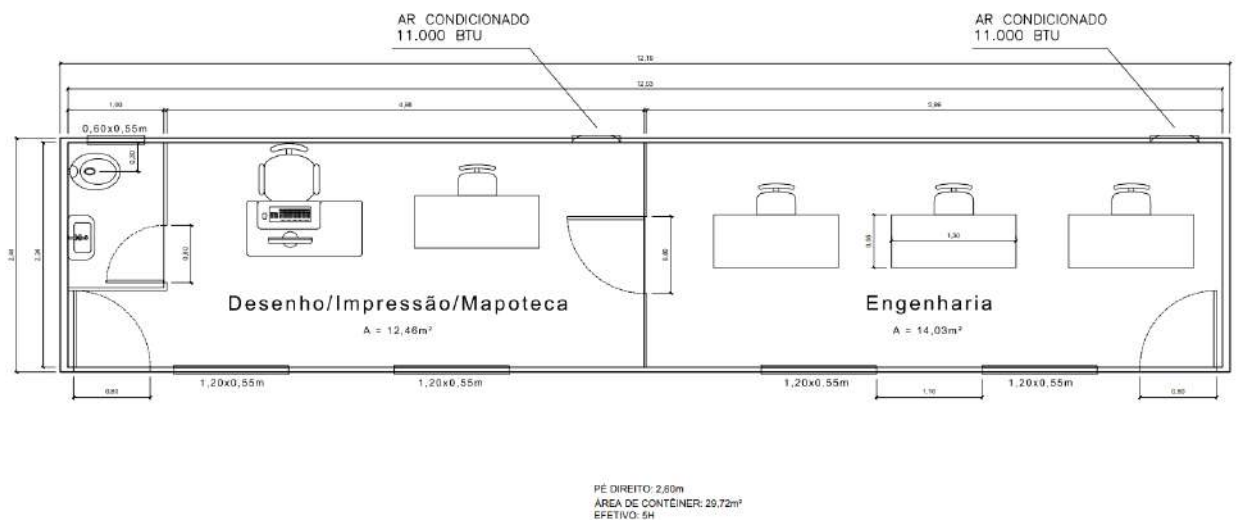
Figura 5 – Seção Técnica – Container 40' (Obras de Pequeno Porte)
