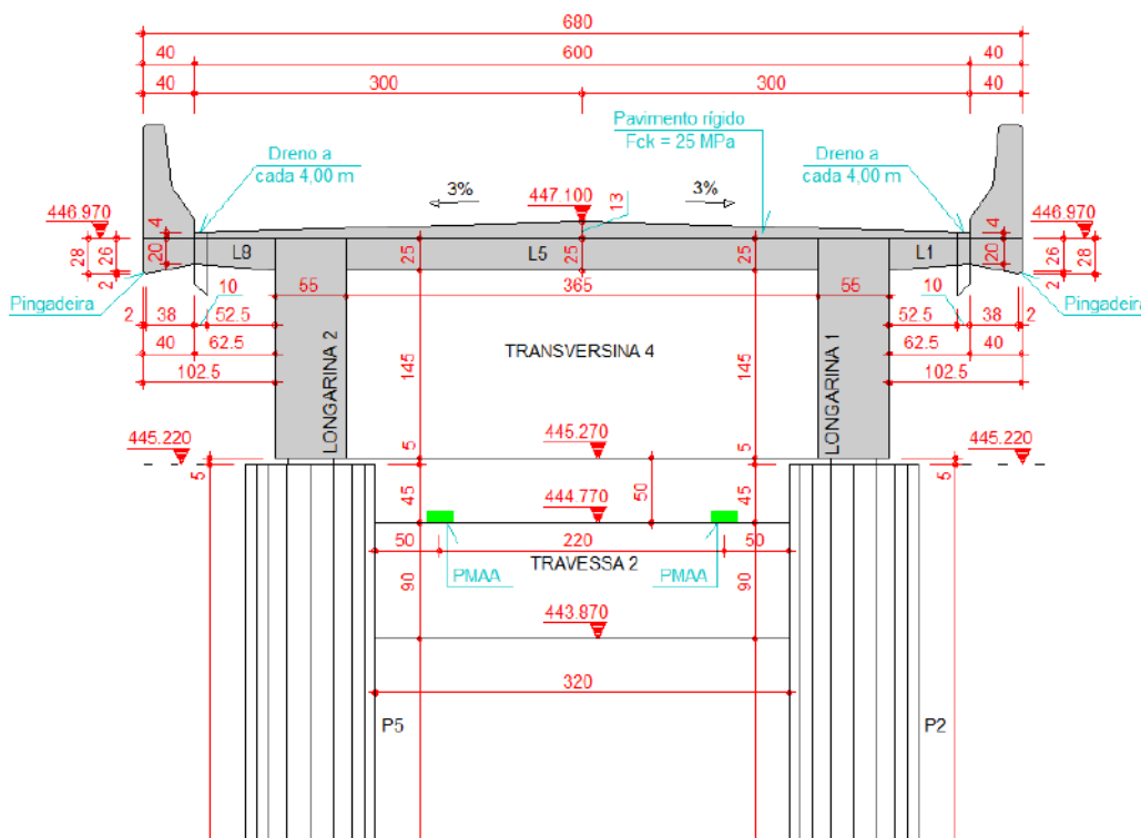
Figura 62 - Corte transversal
