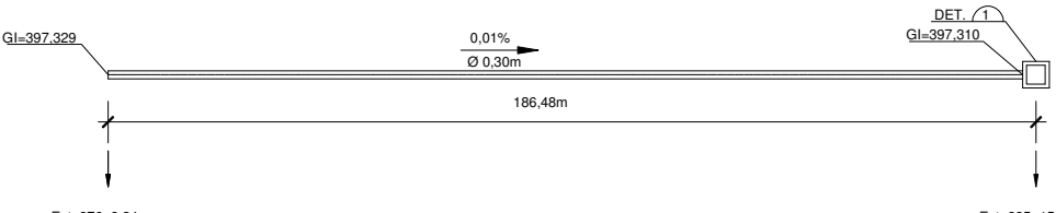
REDE DE DRENAGEM - PERFIL LONGITUDINAL SEM ESCALA
