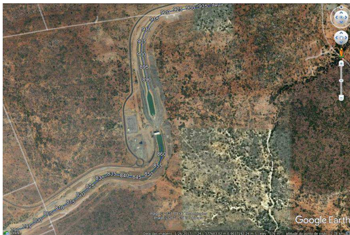
Figura 01: Estação de Bombeamento EBV-2 (WBS 2620), Eixo Leste do PISF.
