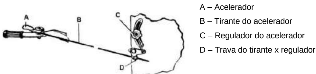
Fig. 6 - Ajuste do sistema de controle e aceleração
