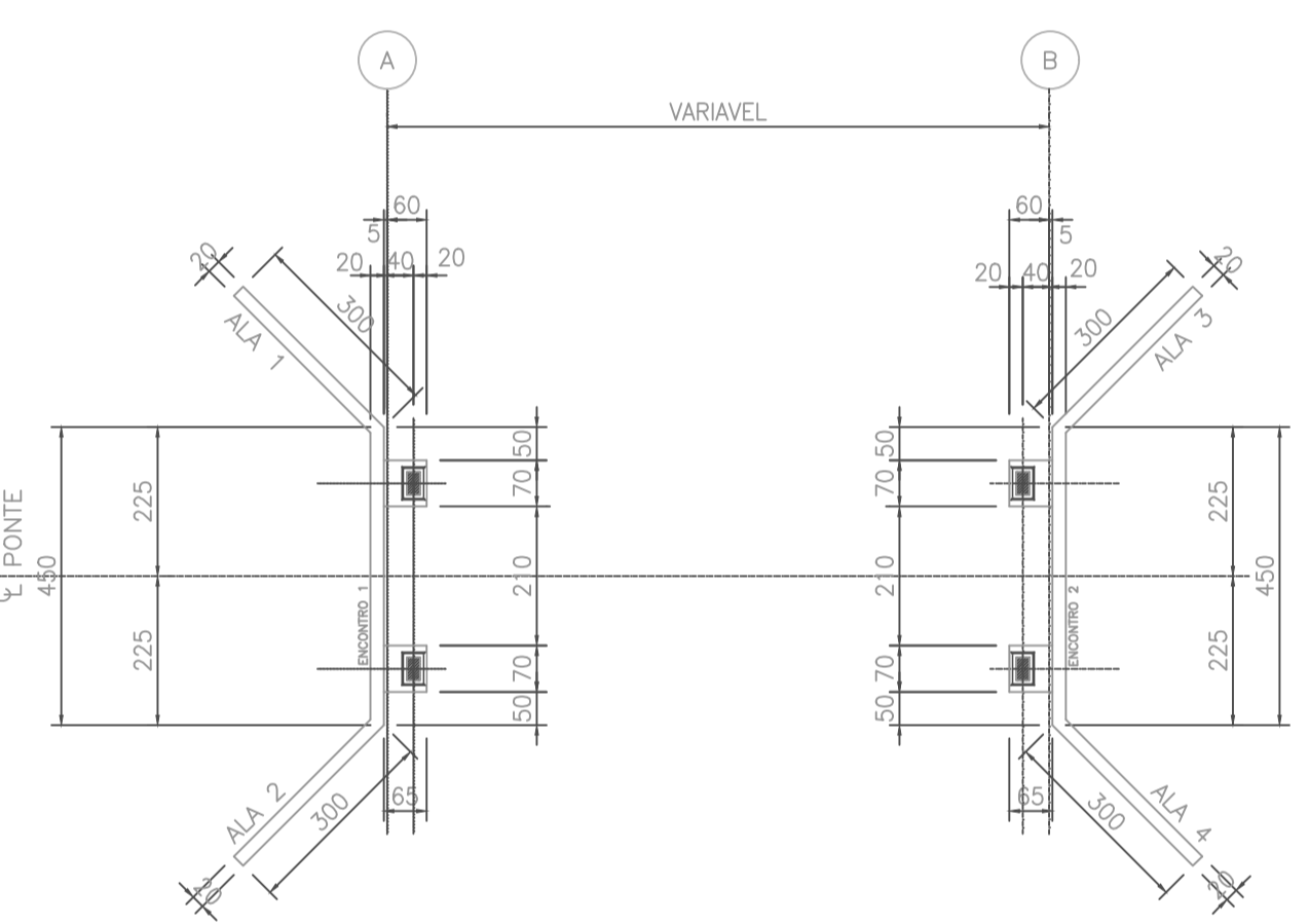
PLANTA DAS FUNDAÇÕES ESC. SEM ESCALA
