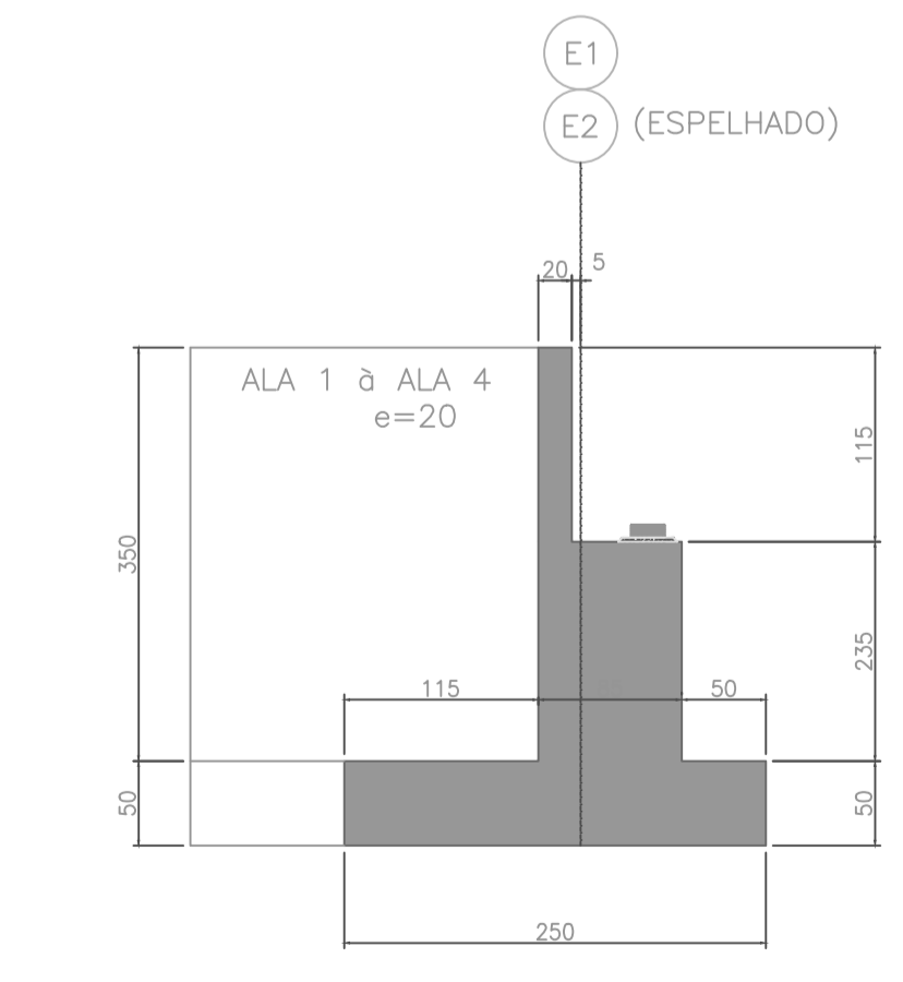
ENCONTROS E1/E2 ESC. SEM ESCALA
